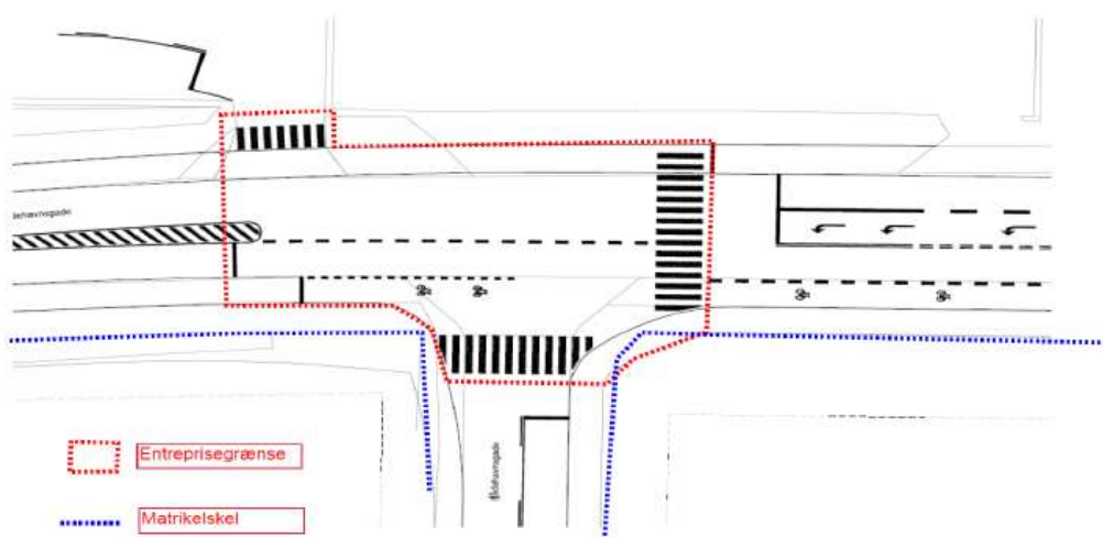
Figur 5-10 – Etablering af lyssignal Mønstertorvet/Bådehavnsvej.
