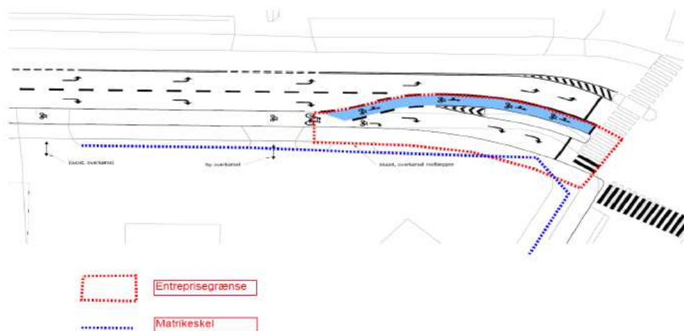
Figur 5-9 – Etablering af cykelbane i krydset Bådehavnsvej/Sjællandsbroen
