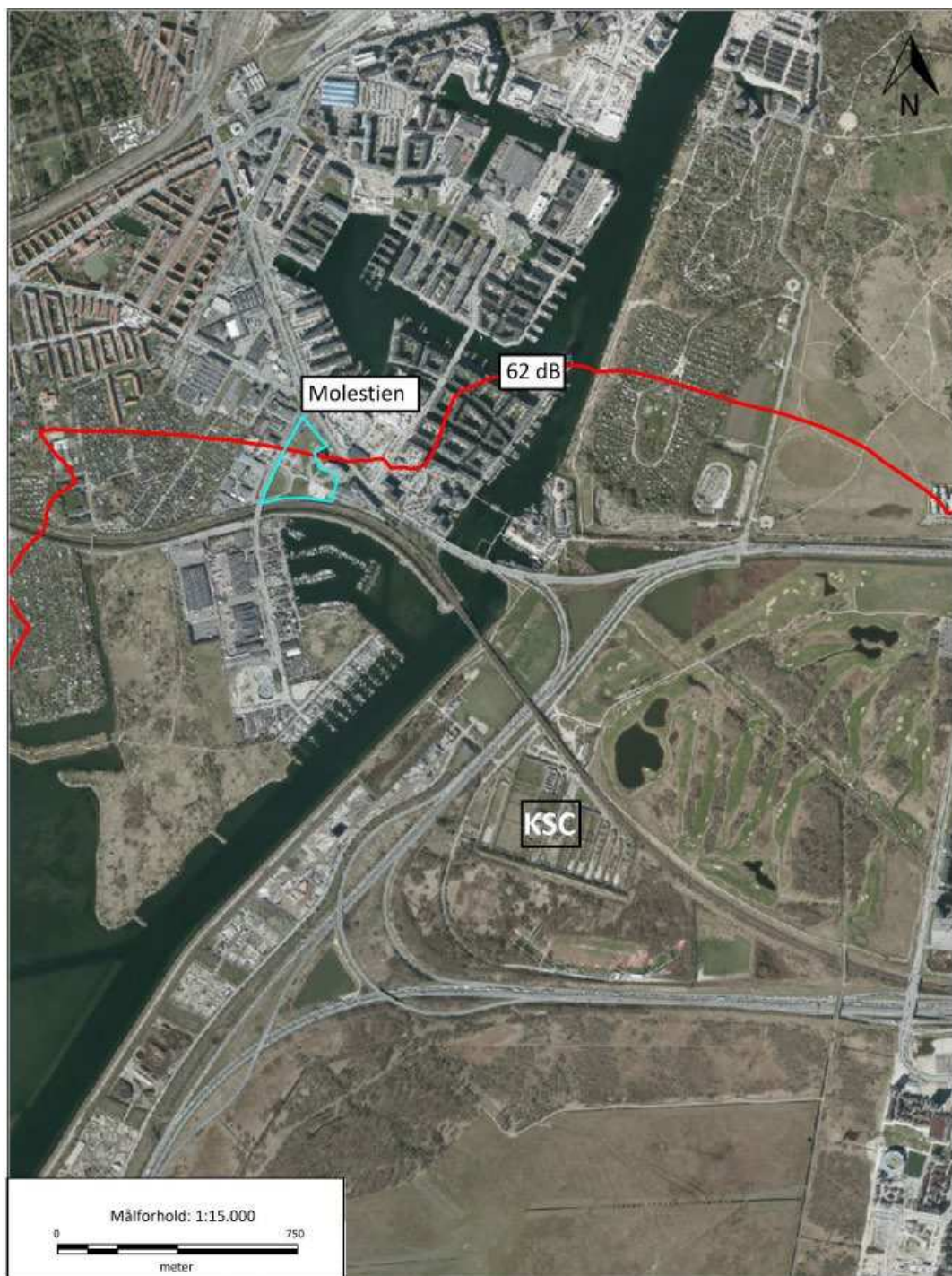
Figur 7-2: Støjudbredelse fra Københavns Skyttecenter (KSC) under eksisterende forhold.
