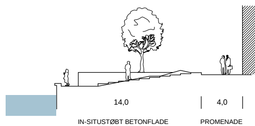
Snit O-O
