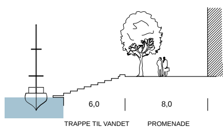
Snit P-P
