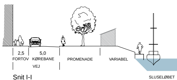
Snit I-I
