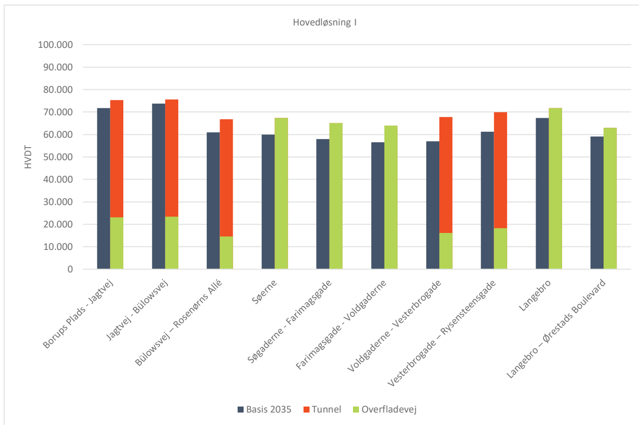
Figur 2-9 Beregnet hverdagsdøgntrafik (HVDT) i 2035 i et basisscenarie og i hovedløsning I på udvalgte snit på strækningen (afrundende tal). Samme tal som anvendt i figur 2-8.
