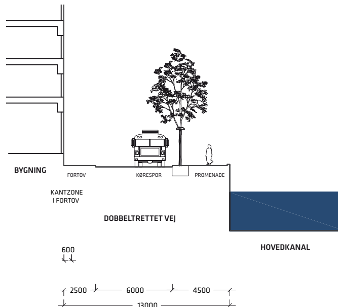
Snit D-D
