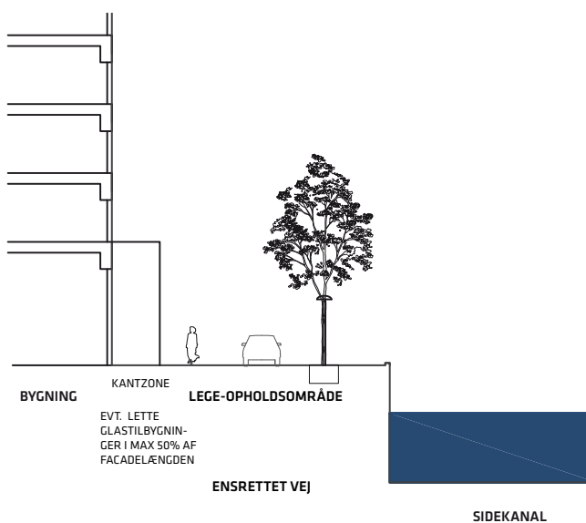
Snit D-D
