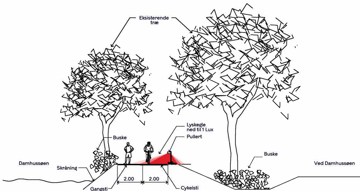
Tværsnit B-B, Projektforslag
