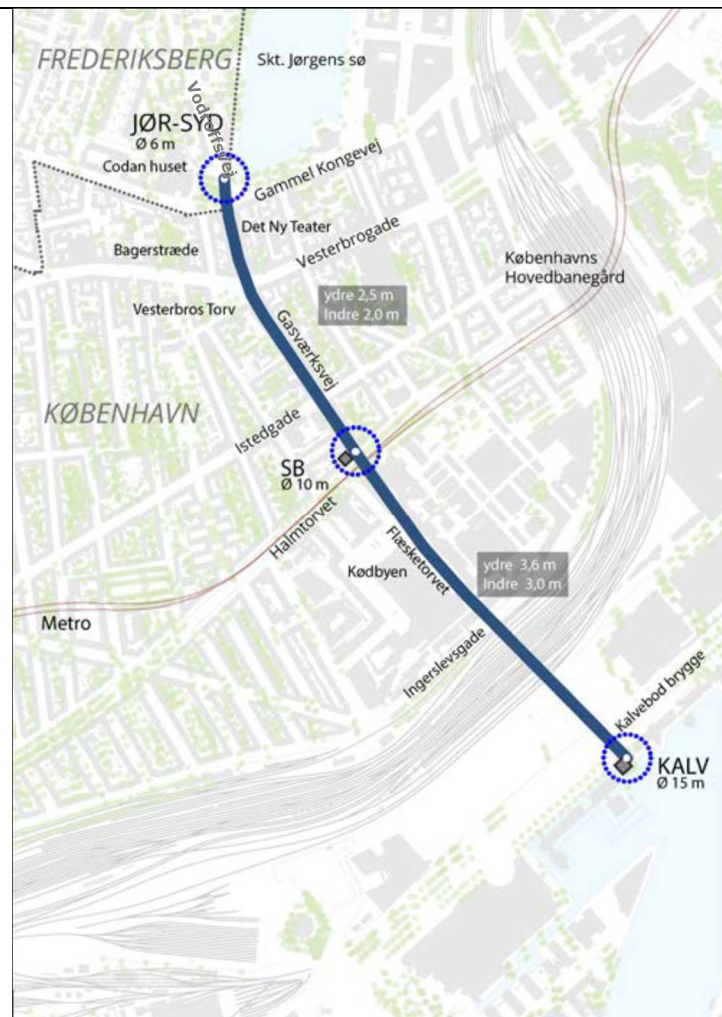
Figur 3.1: Oversigt over placering af skybrudstunnel og bygværkerne JØR-SYD, SB og KALV
