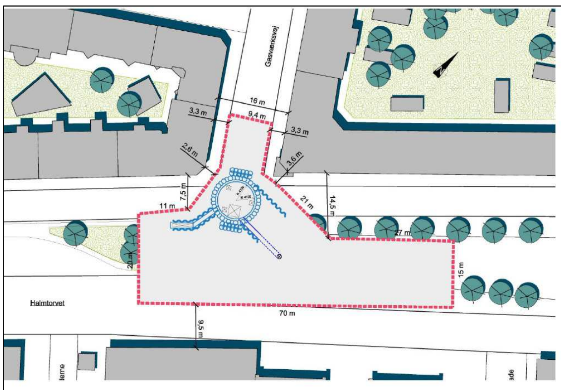
Afgrænsning af byggeplads Lokaltet for kommende byggeskakt SB, fase 2 (etablering af skakt) Rød linje angiver den overordnede byggepladsafgrænsning i perioden.
