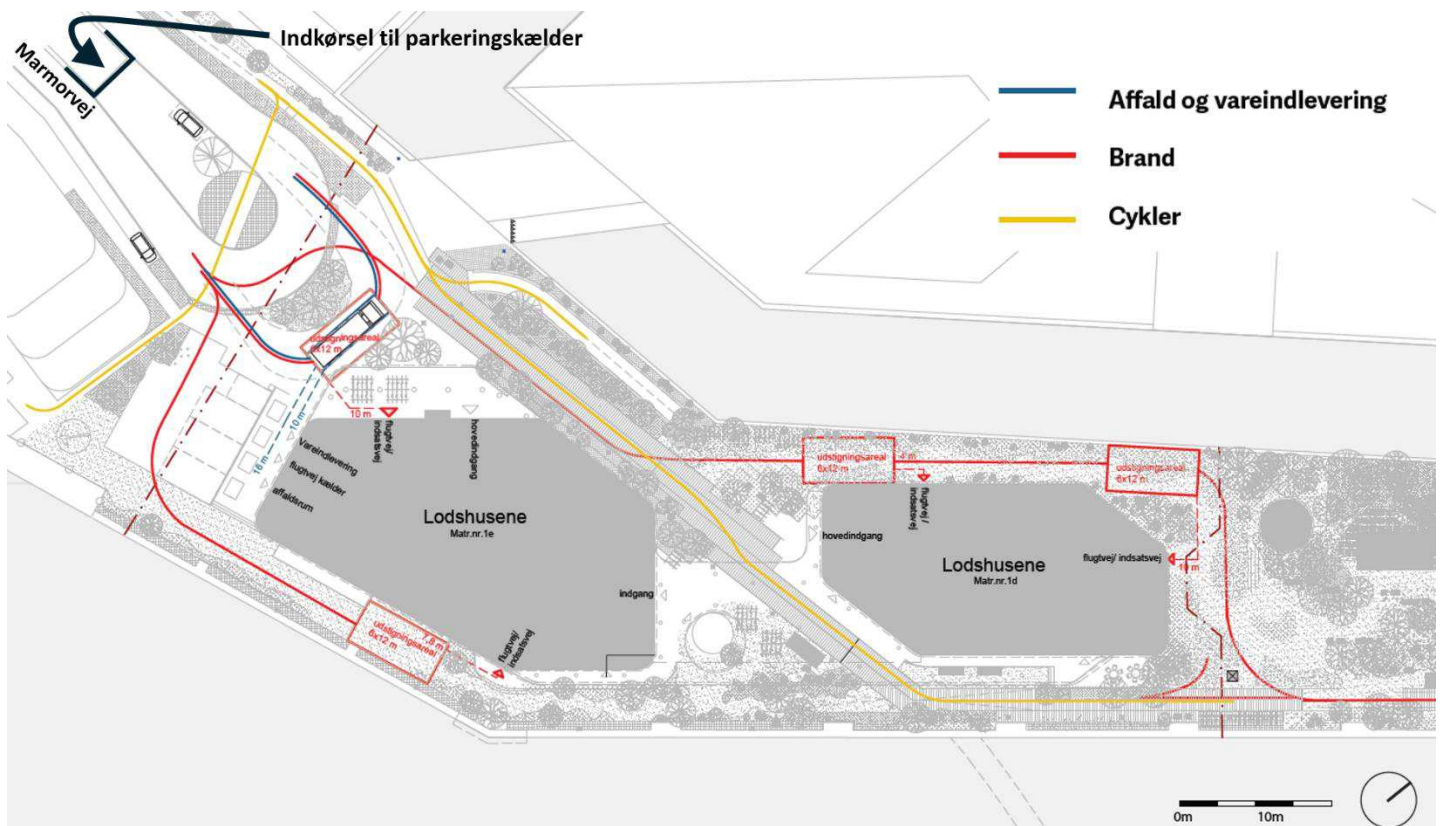
Figur 8-4. Vejadgang til Marmormolen og til underjordisk parkeringsanlæg. VLA, 2025.
