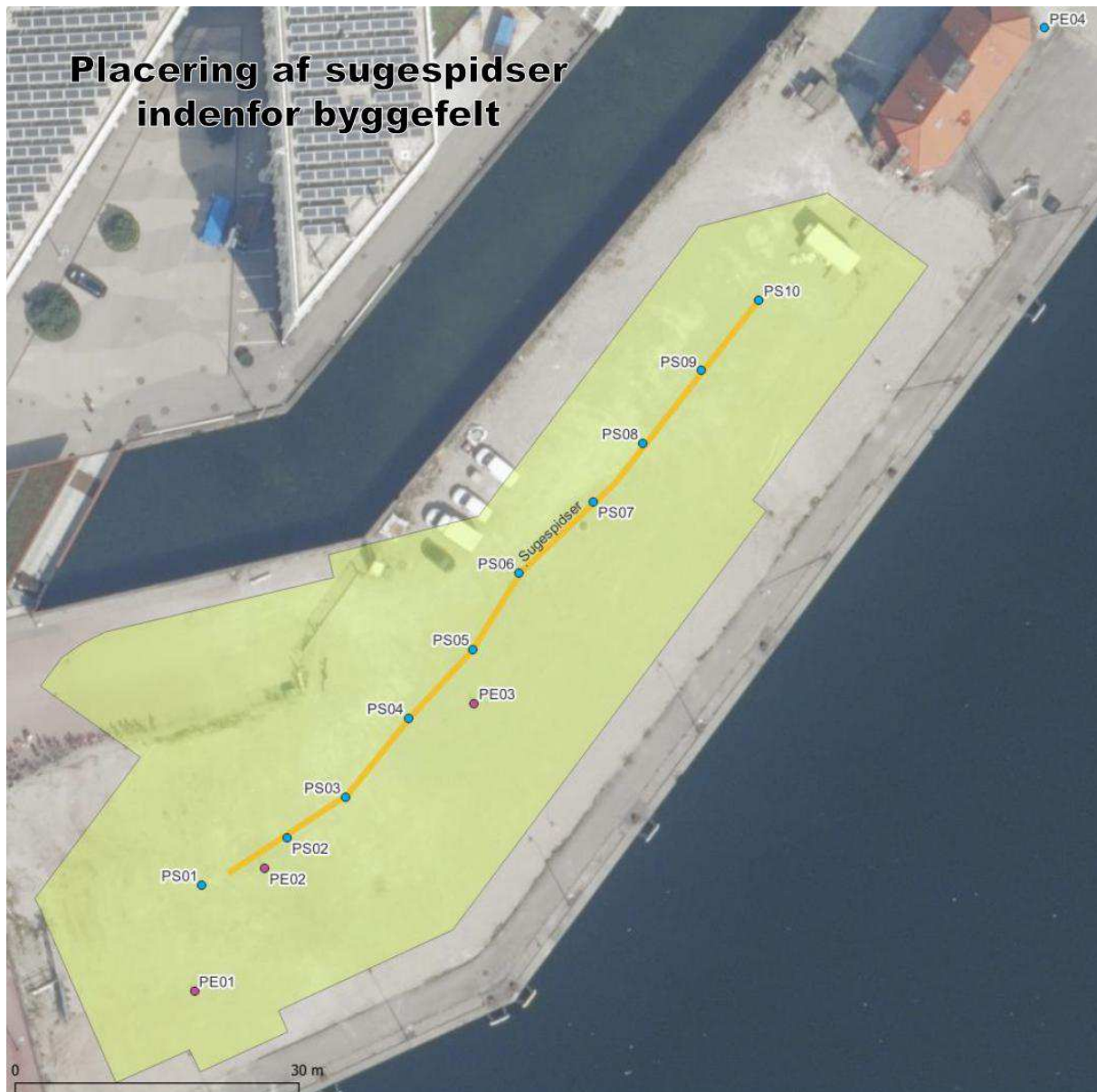
Figur 11-6. Oversigtskort for prøvepumpning. Linje med placering af 40 stk. sugespidsler med ca. 2 m mellemrum er vist med orange streg. 10 stk. af sugespidslerne er taget ud og anvendt som pejlespidsler. Disse er navngivet PS01 – PS10. Pejleboringerne PE01-PE04 er tidligere udførte boringer, der er genanvendt til pejling under forsøget (DMR, 2025).
