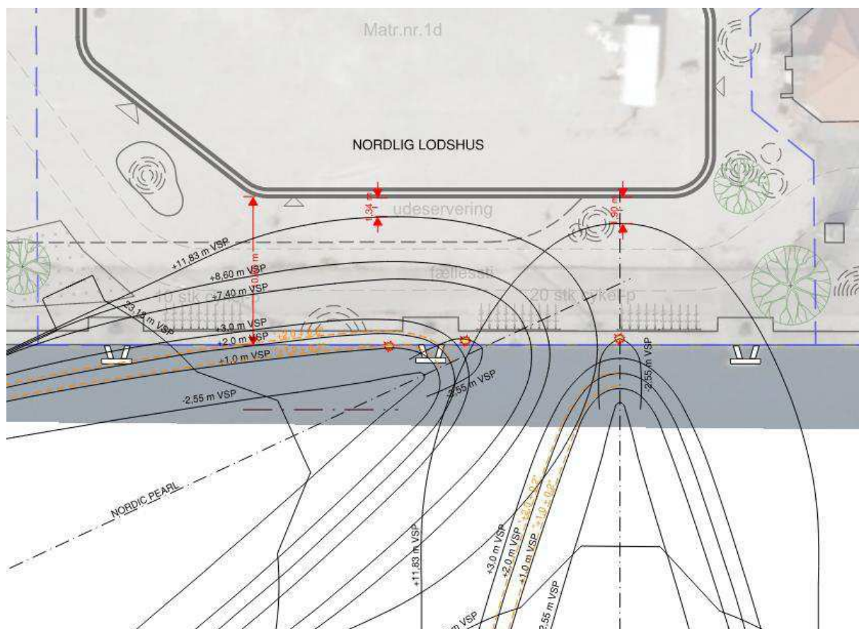
Figur 16-2. Nordligt Lodshus. Nordic Pearl. fendere sejles af og færge støder ind i betonkant med værst mulige vinkel til kaj. Situation til højre viser en frontal påsejling hvor minimumsafstanden bliver ca. 1,9 m. Denne påsejling er kun teoretisk og ikke mulig geometrisk. Situation til venstre viser en påsejling med den vinkel mellem færge og kaj, der giver den mindste afstand mellem færge og lodshus. Mindsteafstanden er her ca. 1,3 m.
