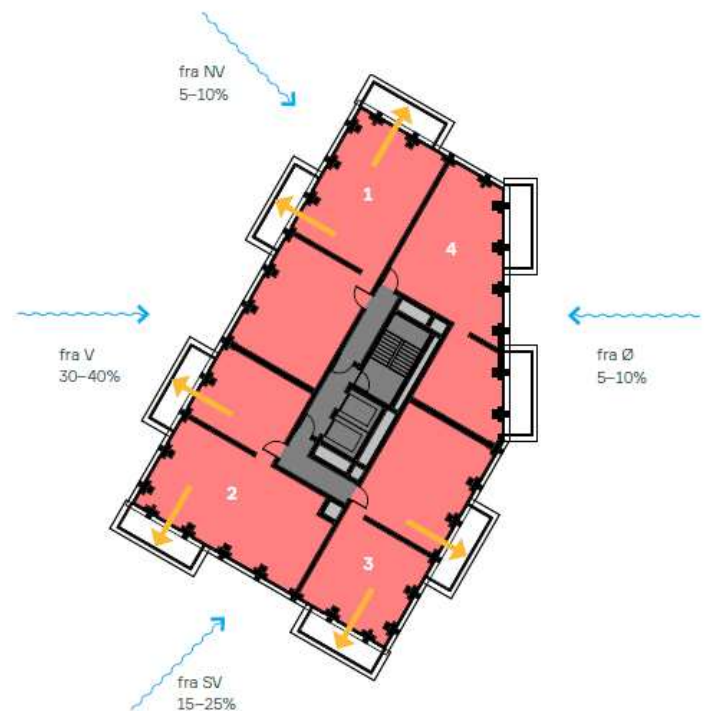
Figur 13-8. Disponering af altaner i to rytmer, der skifter fra etage til etage. Vindretningernes hyppighed angivet med procenttal. Pile inde fra lejligheder angiver mulighed for at tilgå altaner mod to verdenshjørner. Lendager, 2026.
