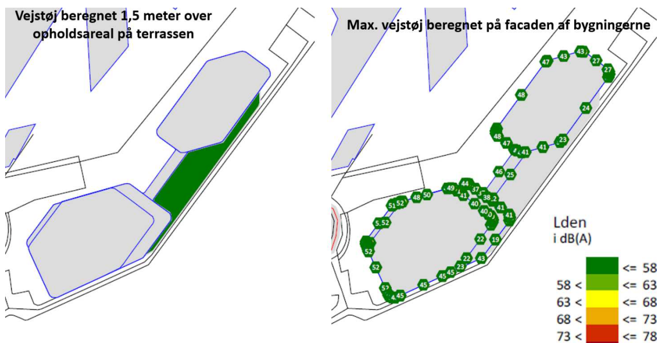
Figur 8-9. Beregnet vejstøj på hhv. opholdsareal på tagterasse og på facaden på Marmormolen. Farvekoder relaterer til grænseværdier i Tabel 8-4.
