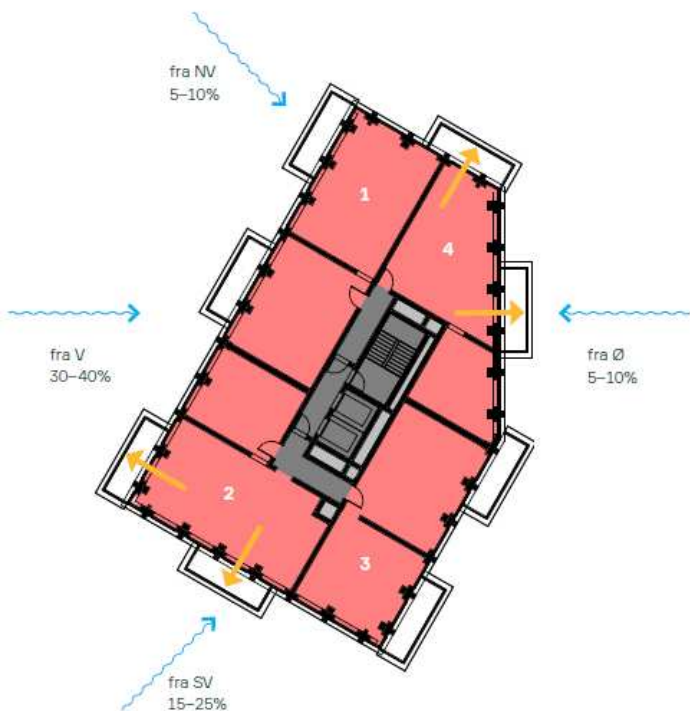
Figur 13-8. Disponering af altaner i to rytmer, der skifter fra etage til etage. Vindretningernes hyppighed angivet med procenttal. Pile inde fra lejligheder angiver mulighed for at tilgå altaner mod to verdenshjørner. Lendager, 2026.
