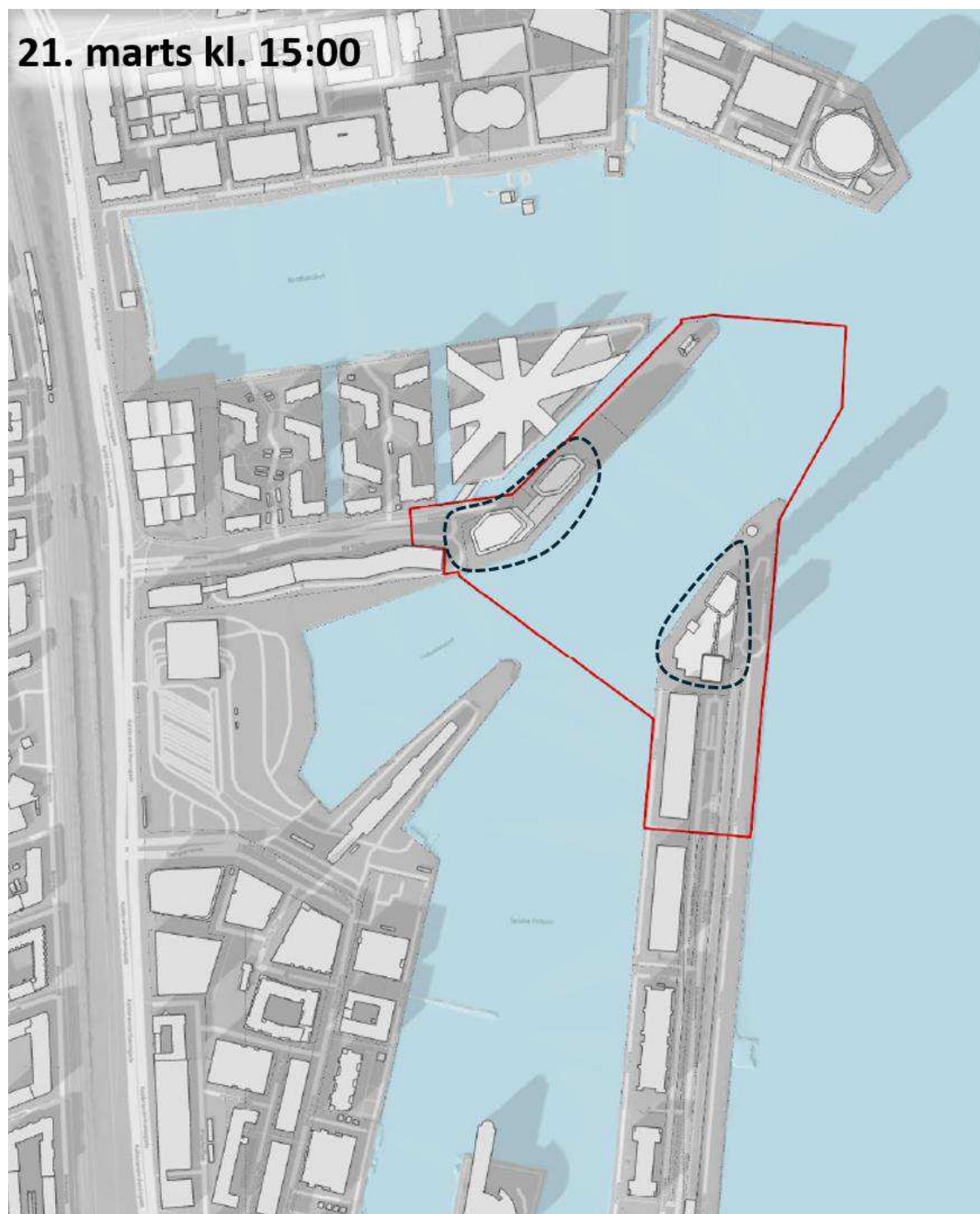
Figur 13-11. Simulering af skyggepåvirkning fra projektet. Projektets bygninger er markeret med stipleet sort linje. Lendager, 2026.
