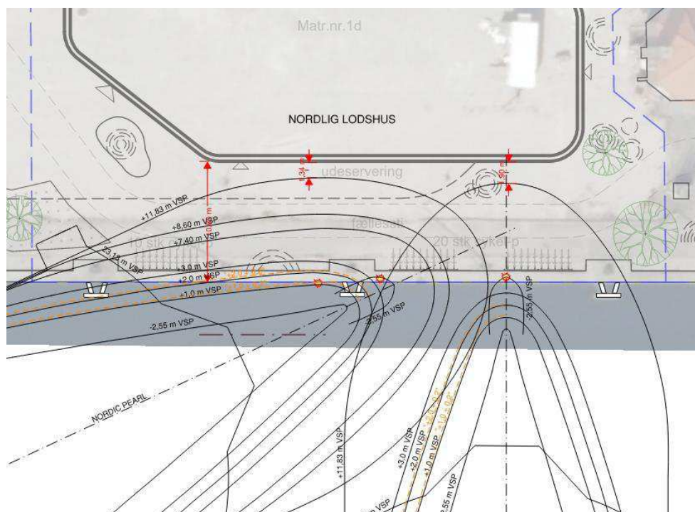
Figur 16-3. Nordlig Lodshus. Nordic Pearl. Fendere sejles af og færge støder ind i betonkant med værste mulige vinkel til kaj. Situation til højre viser en frontal påsejling hvor minimumsafstanden bliver ca. 1,9 m. Denne påsejling er kun teoretisk og ikke mulig geometrisk. Situation til venstre viser en påsejling med den vinkel mellem færge og kaj, der giver den mindste afstand mellem færge og lodshus. Mindsteafstanden er her ca. 1,3 m.
