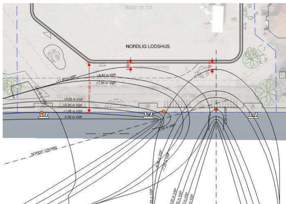
Figur 16-4. Nordlige Lodshus. Nordic Crown. Fendere sejles af og færge støder ind i betonkant med værste mulige vinkel til kaj. Situation til højre viser en frontal påsejling, hvor minimumsafstanden bliver ca. 1,3 m. Denne påsejling er kun teoretisk og ikke mulig geometrisk. Situation til venstre viser en påsejling med den vinkel mellem færge og kaj, der giver den mindste afstand mellem færge og lodshus. Mindsteafstanden er her ca. 0,9 m.
