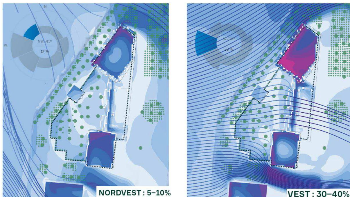
Figur 9-8. Simulering af vindpåvirkning på facader fra de fire fremherskende vindretninger. Farveskala for vindhastigheds indsat. Byggefelt markeret med stiplede linje. Lendager, 2026.
