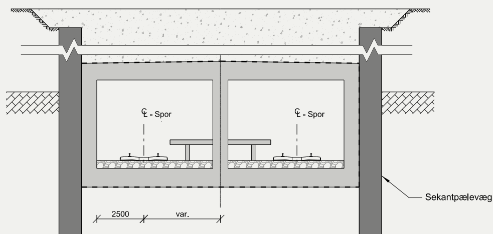
Figur 7.5: Typisk tværsnit i cut og cover-tunnel.
