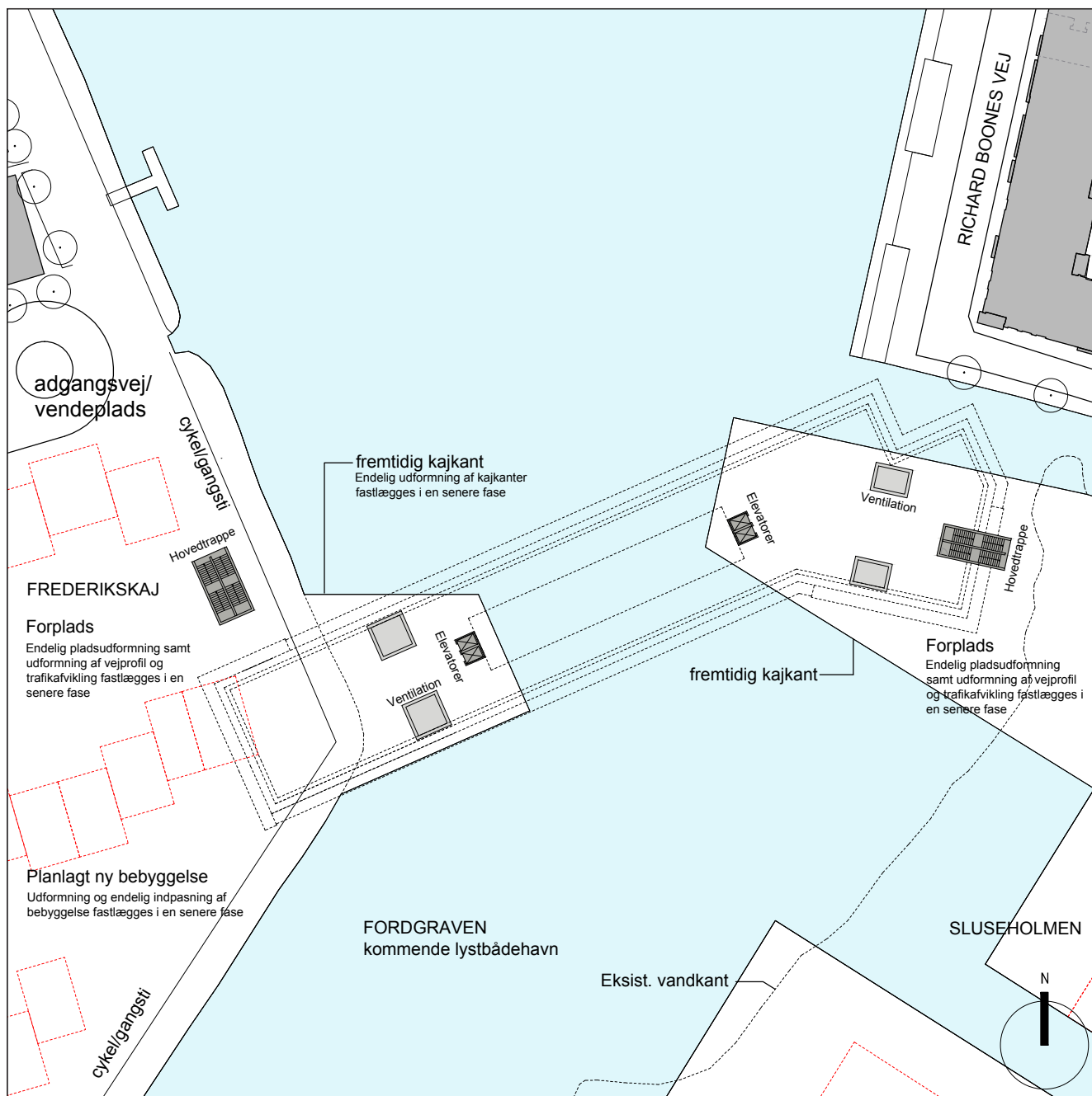
Figur 6.20: Forslag til stationsplacering af v/Slusen. Stationen er vist som en kanalstation med elevatorer, trapper og ventilation. Figuren kan ses i 1:1.000 i tegningsbilaget.
