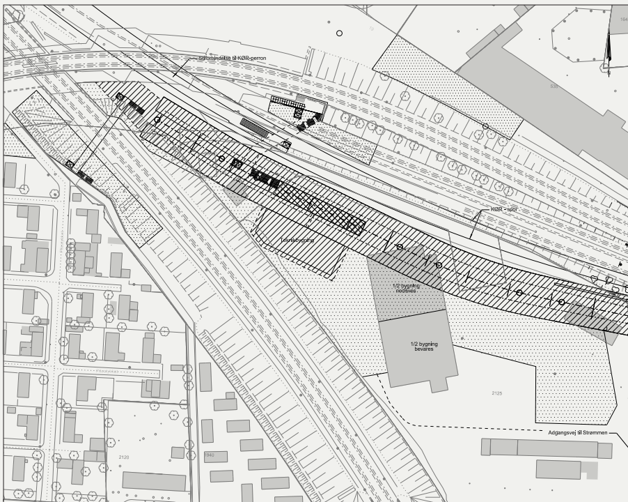
Figur 7.19: Forslag til arbejdspladsudformning for Ny Ellebjerg station på terræn. Figuren kan ses i 1:1.000 i tegningsbilaget.
