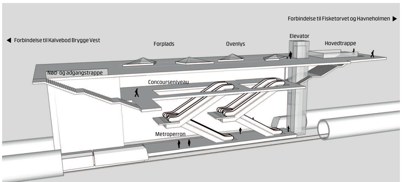
Figur 6.8: 3D-illustration af v/Fisketorvet. Stationen er vist som en undergrundsstation med gennemgående concoursniveau.
