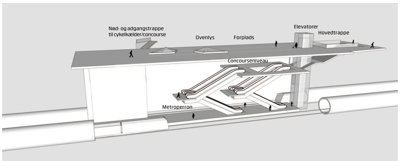
Figur 6.30: 3D-illustration af v/Mozarts Plads. Stationen er vist som en undergrundsstation med terræn-, concourse- og perronniveau.
