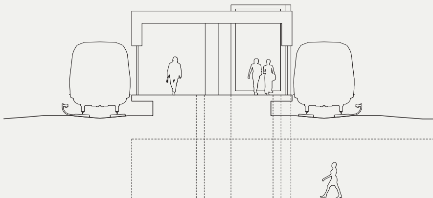
Figur 6.6: Tværsnit af en station på terræn.
