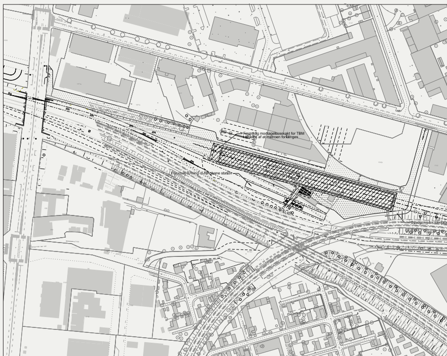
Figur 7.20: Forslag til arbejdspladsudformning for Ny Ellebjerg, undergrundsstation.
