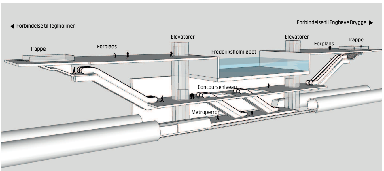
Figur 6.14: 3D-illustration af v/Frederiksholmsløbet station. Stationen er vist som en kanalstation med terræn-, kanal-, gennemgående concourse- og perronniveau.
