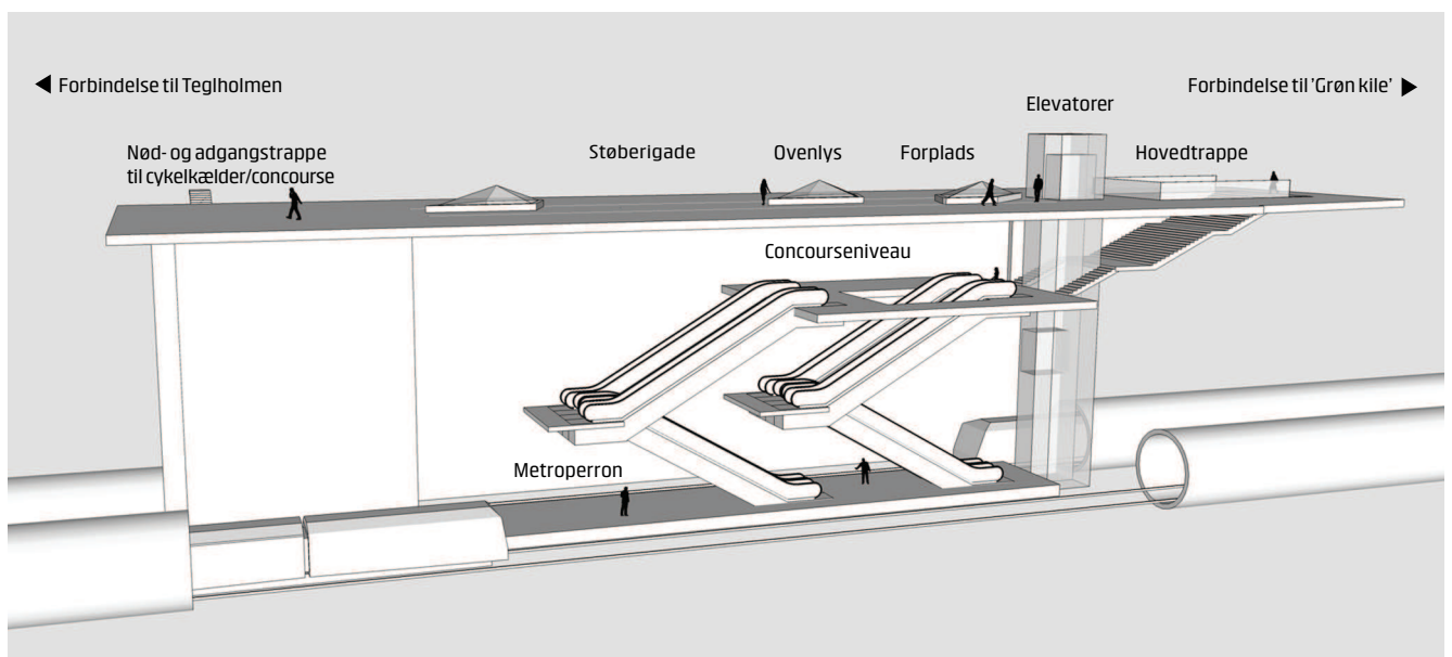
Figur 6.18: 3D-illustration af v/Teglholmen. Stationen er vist som en undergrundsstation med terræn-, concourse- og perronniveau.
