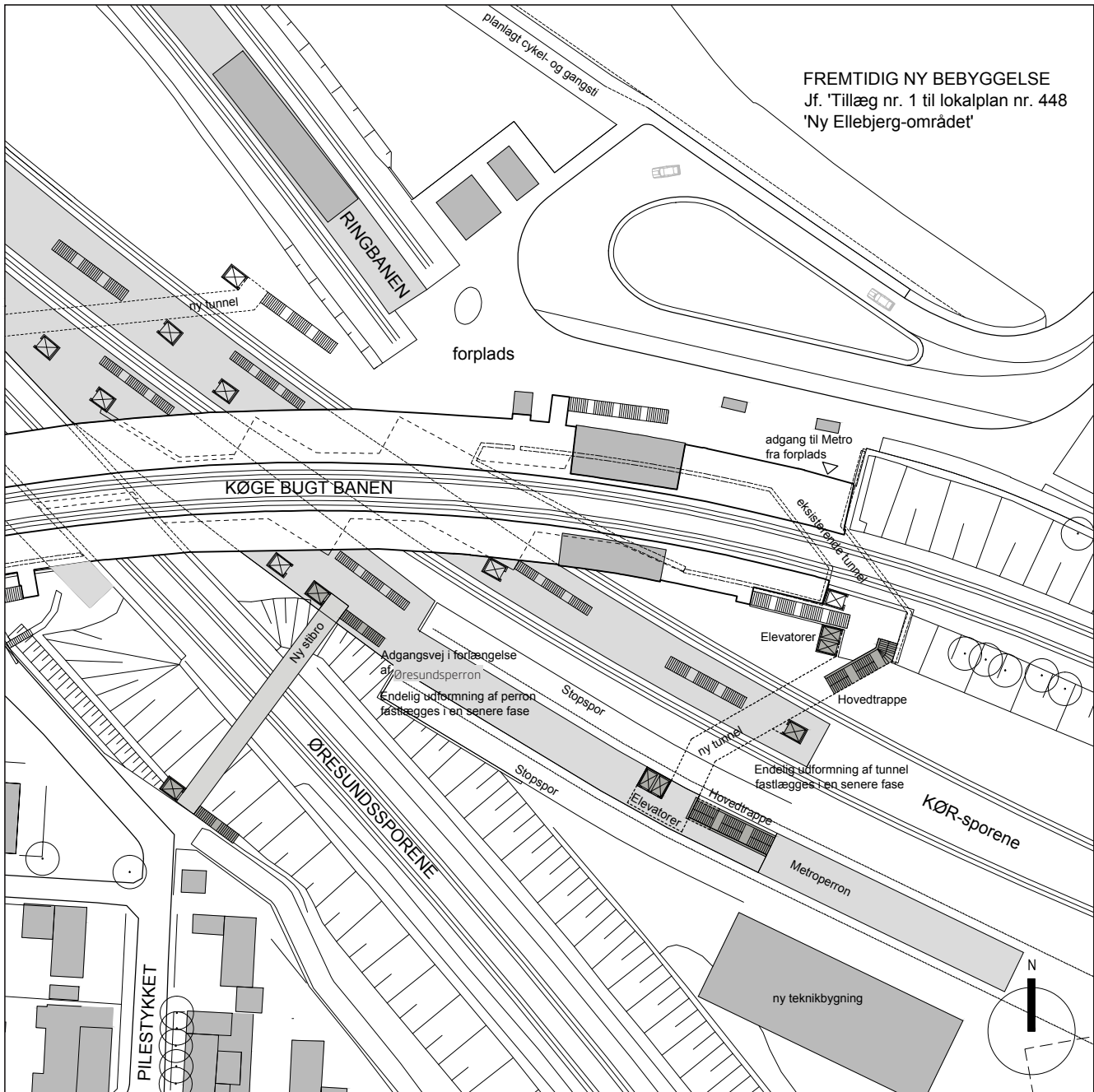
Figur 6.32: Forslag til stationsplacering af Ny Ellebjerg station på terrænen. Stationen er vist som en station på terrænen med elevatorer og trapper. Figuren kan ses i 1:1.000 i tegningsbilaget.
