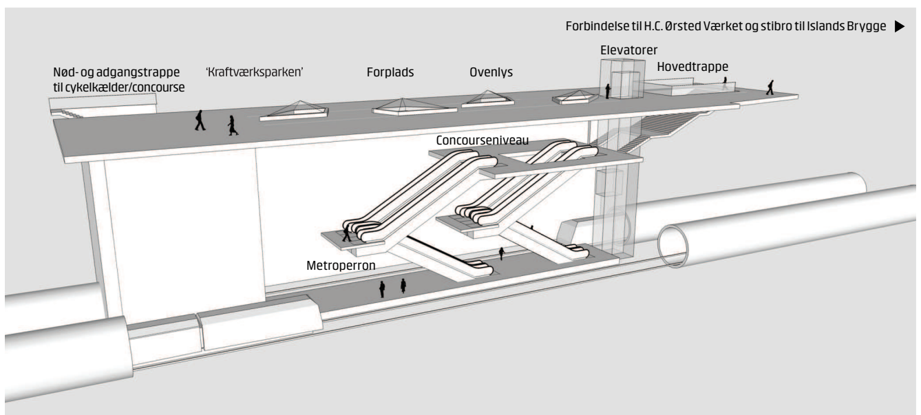
Figur 6.11: 3D-illustration af v/Enghave Brygge. Stationen er vist som en undergrundsstation med terræn-, concourse- og perronniveau.
