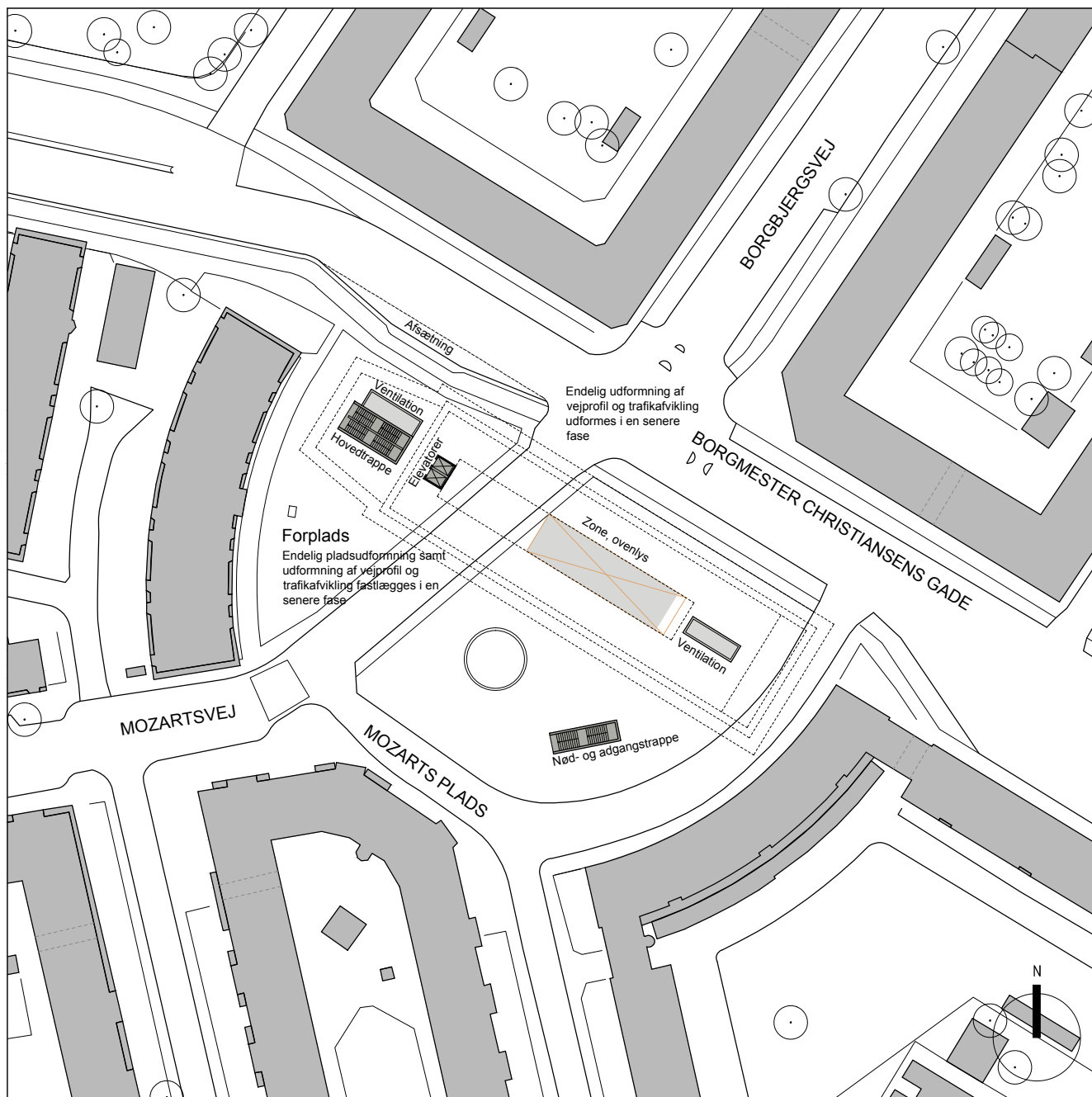
Figur 6.29: Forslag til stationsplacering af v/Mozart Plads (undergrundsstation). Stationen er vist som en undergrundsstation med elevatorer, trapper og ventilation. Figuren kan ses i 1:1.000 i tegningsbilaget.
