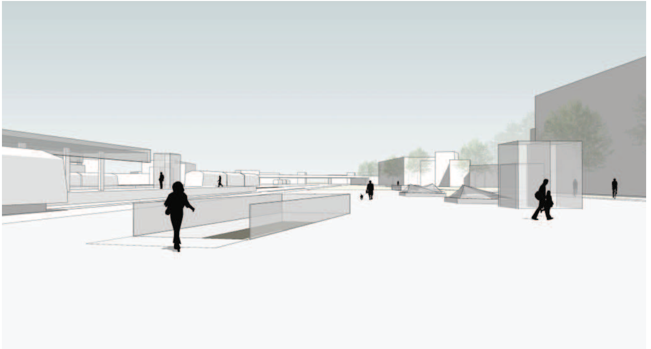
Figur 6.38: 3D-perspektiv af Ny Ellebjerg som undergrundsstation. Stationen er vist fra forpladsen med trappenedgang og elevator i forgrunden og den øvrige station i baggrunden.
