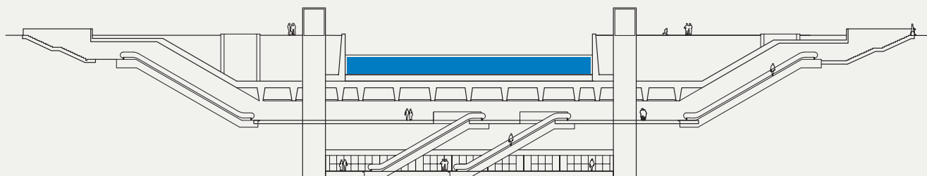
Figur 6.4: Længdesnit af en kanalstation.
