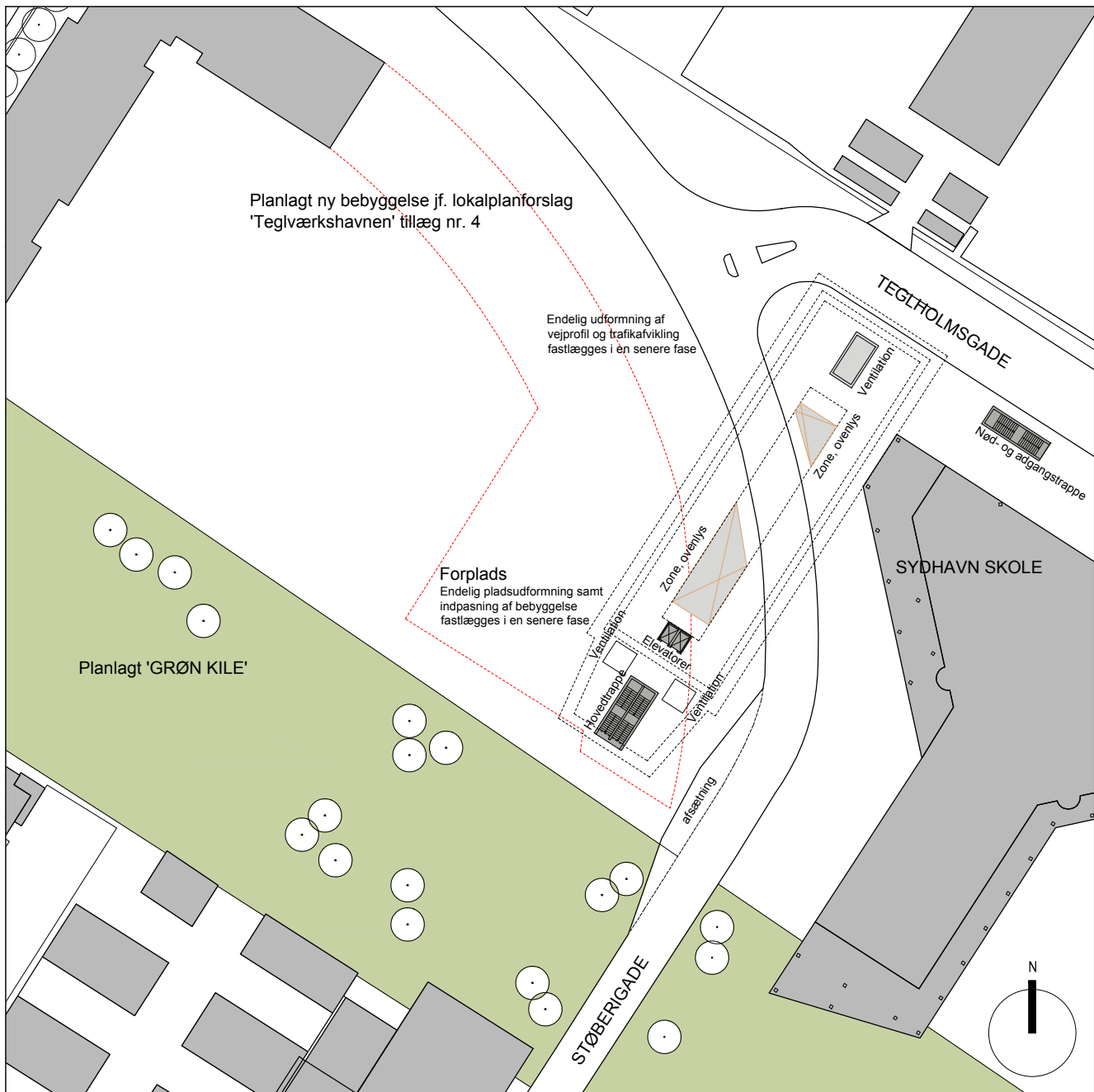
Figur 6.17: Forslag til stationsplacering af v/Teglværksholmen. Stationen er vist som en dyb undergrundsstation med elevatorer, trapper og ventilation. Figuren kan ses i 1:1.000 i tegningsbilaget.
