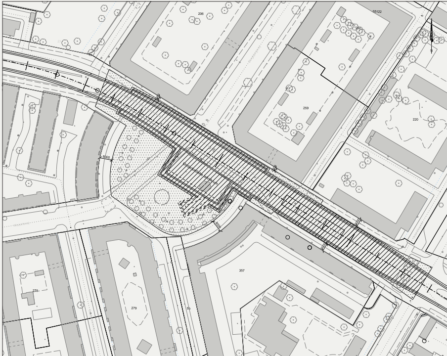
Figur 7.17: Forslag til arbejdspladsudformning for v/Mozarts Plads (åben grav). Figuren kan ses i 1:1.000 i tegningsbilaget.
