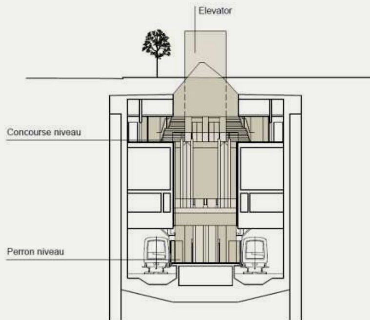
Figur 6.3: Tværsnit af en undergrundsstation, Nuuks Plads.
