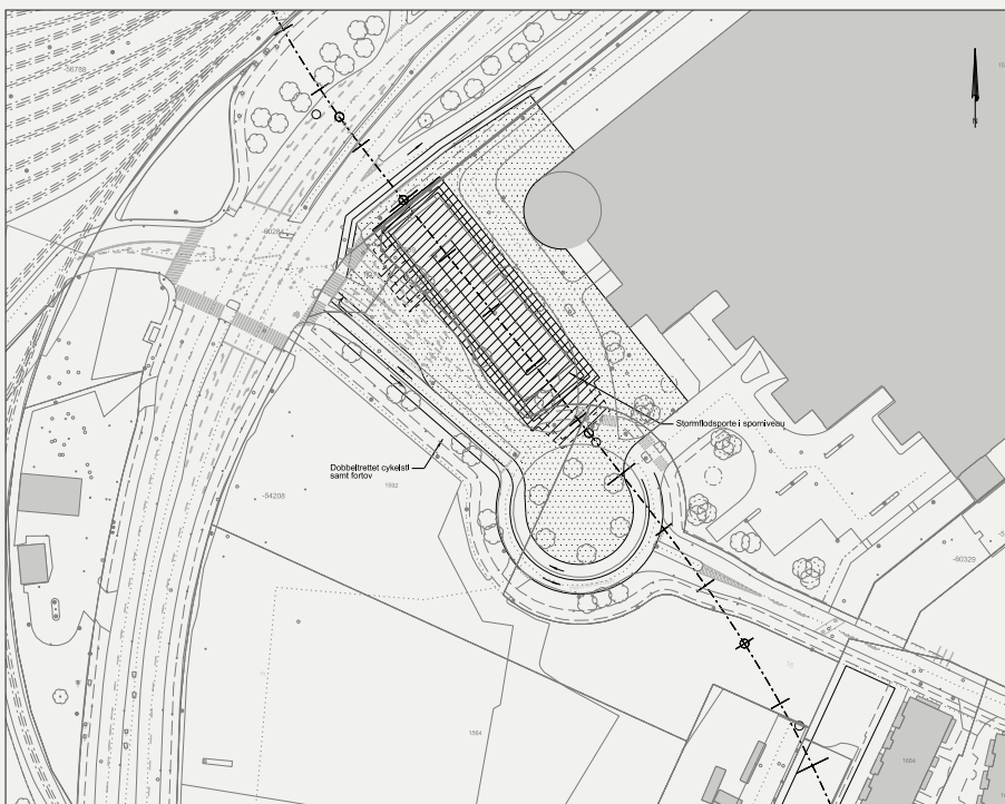
Figur 7.13: Forslag til arbejdspladsudformning for v/Fisketorvet. Figuren kan ses i 1:1.000 i tegningsbilaget.
