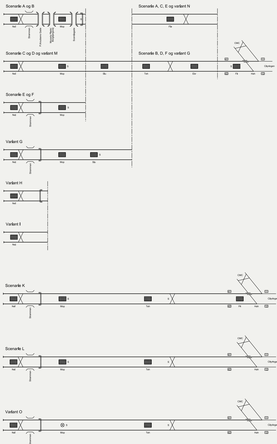
Figur 7.3: Schematisk sporplan visende Sydhavnsmetroen scenarier og varianter inkl. Sydhavnsmetroens tilslutning til Cityringen i Havneholmen afgreningskammer.
