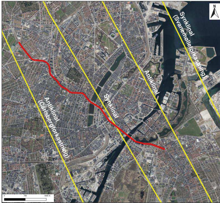
Figur 7-8 Geologiske strukturer i projektområdet, modificeret fra [8]. Den østligste synklinal udgør Svanemølleforkastningen, den vestligste synklinal er orienteret under Rådhusdalen og den vestligste anfklinal udgør Carlsbergforkastningen. Den Grønne Boulevard er angivet med rød linje.
