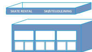
Isometri af skøjteudlejning Mål udv. total: Længde 5,9 meter Bredde 2,34 meter Højde: 2,28 meter
