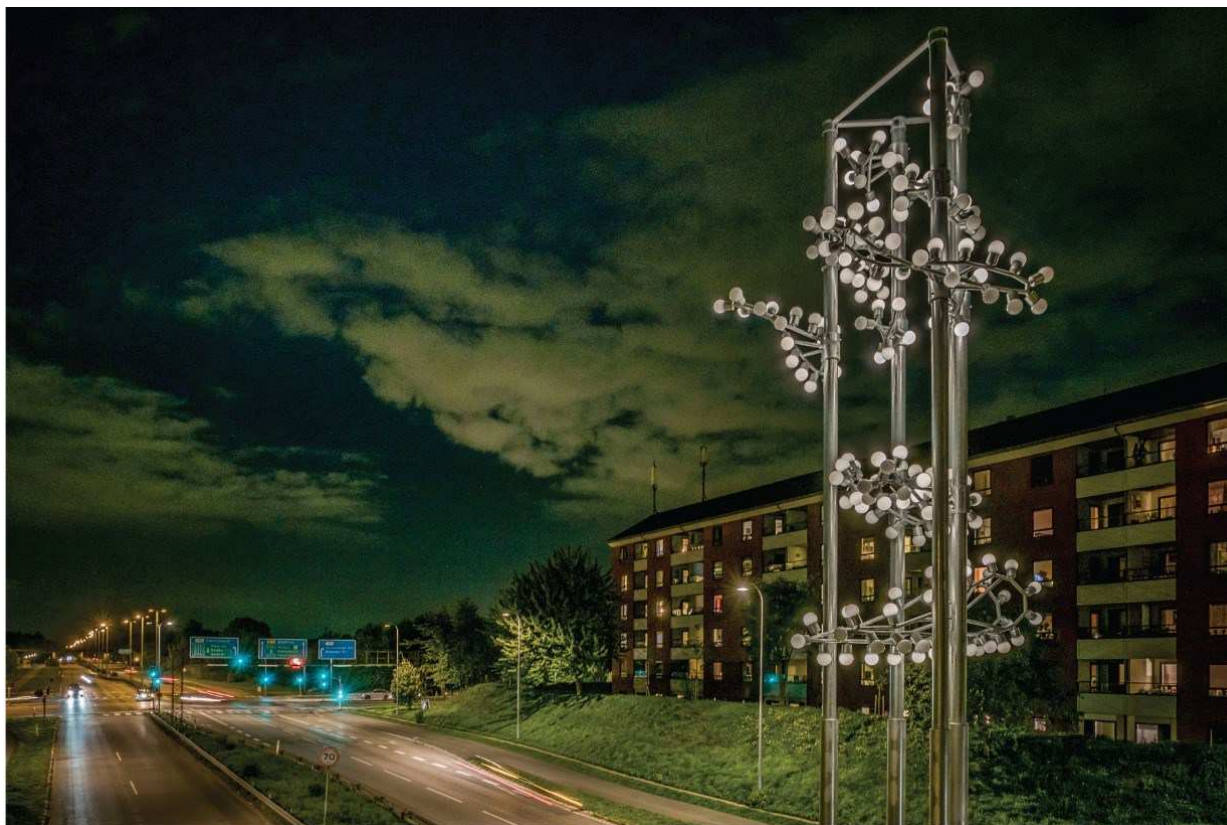
Gænger, 2018. Permanent udendørs installation i Vallensbæk. Stålmaster, glaskupler, LED-lys, PLC, DMX-kontrol, mikrobølge-radar. 3,7 m x 3,5 m x 13,5 m
