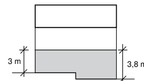
Stueetage med split level
