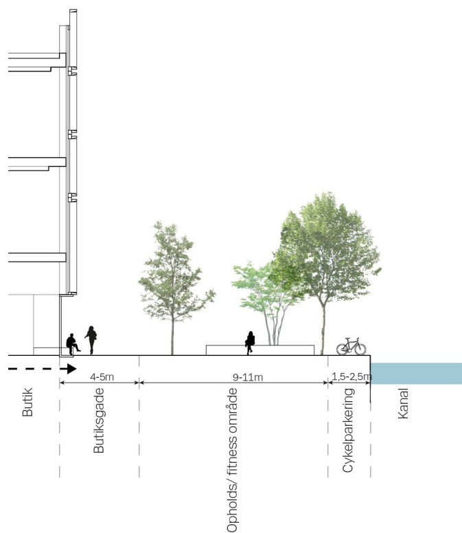
Snit B-B
