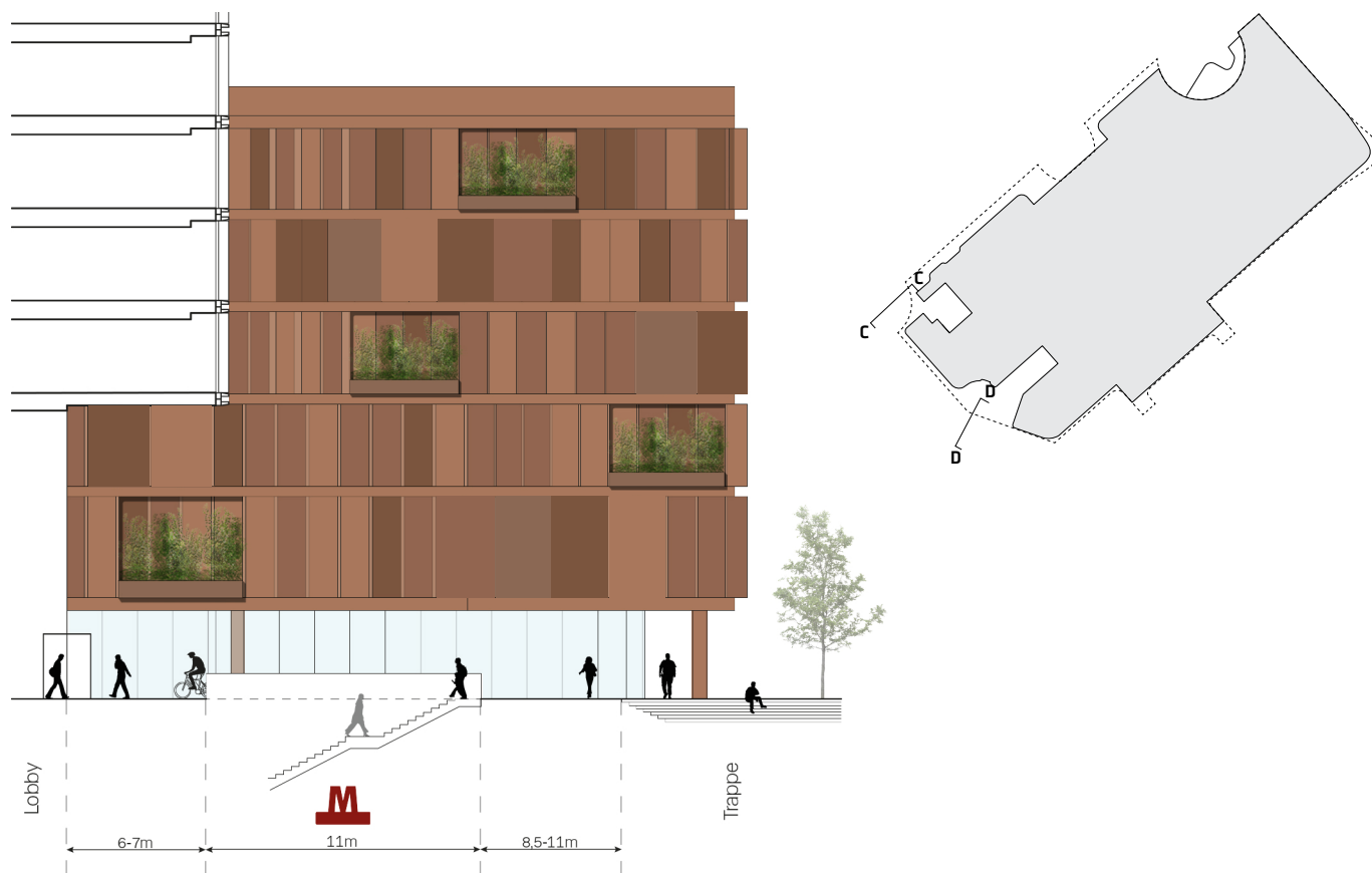
Snit C-C
