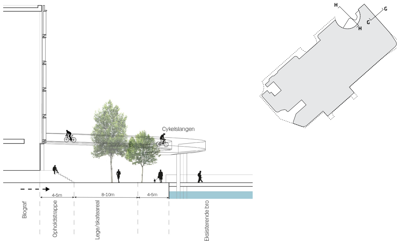
Snit G-G
