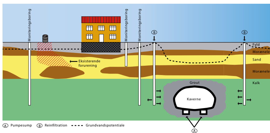
Figur 15.7 Princip for grundvandskontrol omkring kaverne
