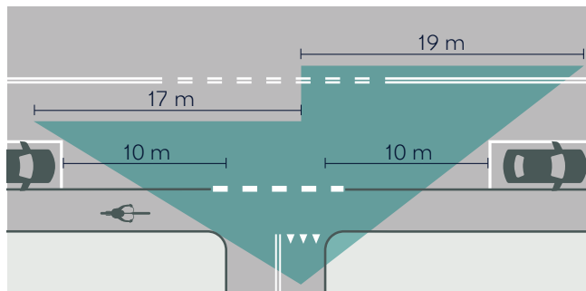
Figur 20: Oversigtsforhold fra sidevejen, med bilparkering 10 m fra krydset
