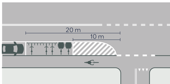
Figur 21: Mellem 10-20 m fra krydset kan der etableres cykelparkering
