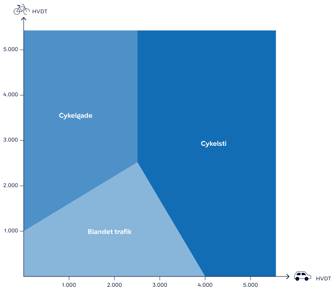
Figur 1 Vejledning til cykelinfrastruktur i sammenhæng med trafikmængder
