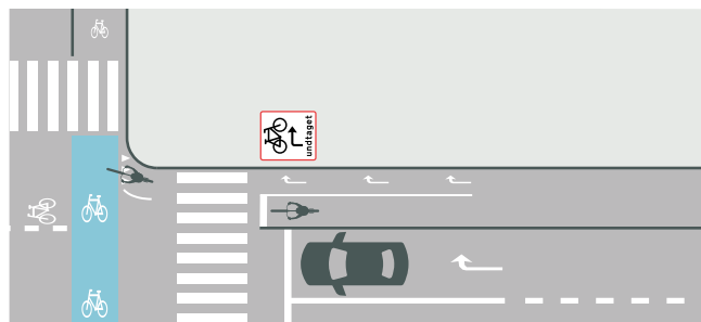
Figur 22: Højresvingende cyklister undtaget signalregulering
