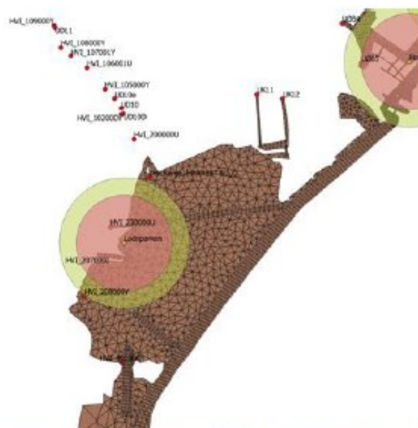
Figur 5 Zoom ind på Lodsparken og Havnebadet Sluseholmen. Ellers som Figur 2. Overløbet HVI_207000I, som løber ud lige syd for Lodsparken er sammenfaldende med 3 andre overløb som ikke fremgår af kortet. Det er HVI_207000U, HVI_207000Y og HVI_207016B.
