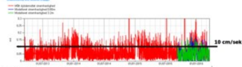
Strømning ved Islands Brygge
