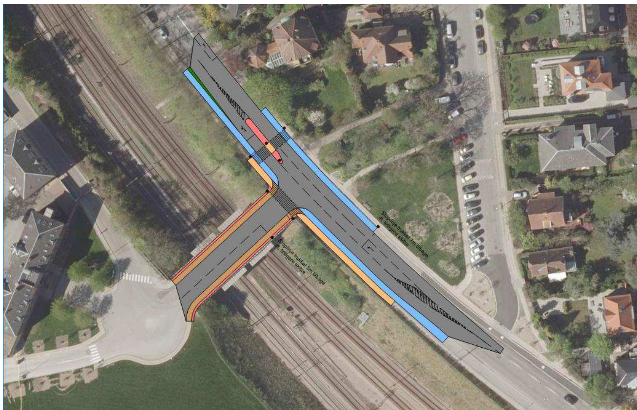
Figur 5-2 Principskitse for løsning med fællesstier i begge sider af vejen. Stopstregen på broen er trukket langt tilbage for at indsvingende lastbiler kan komme rundt.
