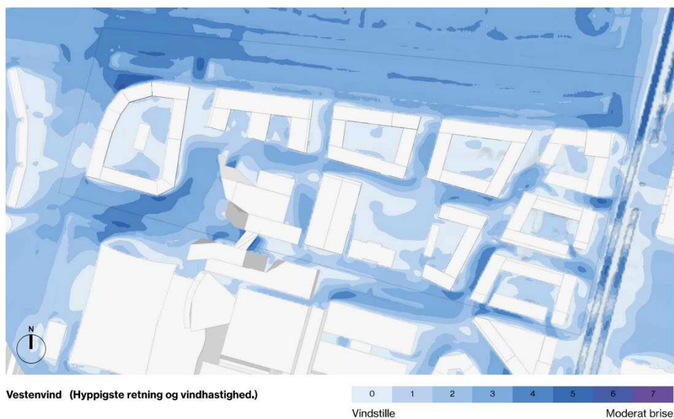
Figur 10-3. Modeller over vindforhold ved det planlagte byggeri inkl. Byggefelternes numre fra bilag 5.
