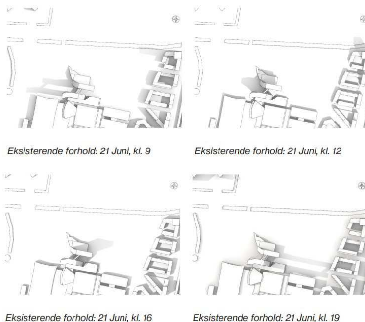
Figur 9-1. Skyggediagrammer for de eksisterende forhold hhv. d. 21. marts og 21. juni.
