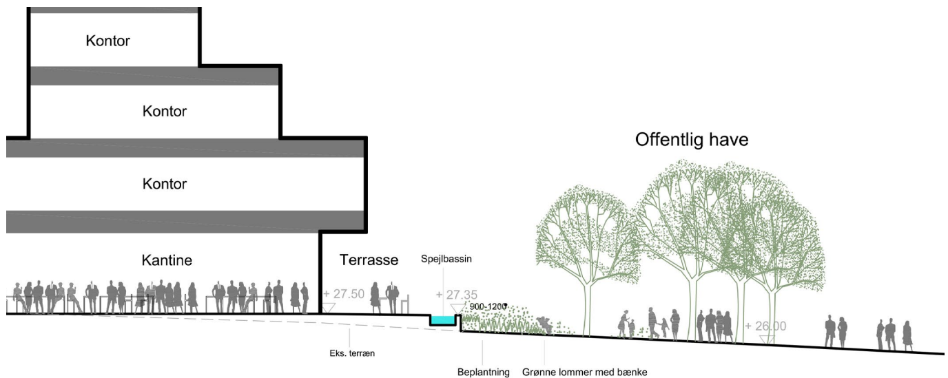
Snit med privat terrasse/kantzone langs hovedsædets stueetage mod haven. En lav beplantning adskiller den offentlige have og den private terrasse. På havesiden etableres lommer med bænke. Med stiplet linje ses det eksisterende terræn i haven. Illustration: C.F. Møller
