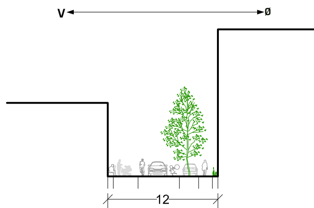
Fig. 4.3. jf. § 4 stk 5, Stræde . Principalsnit af et stræde
