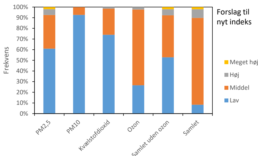
Figur 2.4. Den procentvise fordeling af de forskellige indeksniveauer ved bybaggrunds-målestationen på taget af H.C. Ørsted Institut i 2021 beregnet på basis af det nye forslag til luftkvalitetsindeks. Figuren inkluderer både et samlet luftkvalitetsindeks beregnet ud fra PM 2,5 , PM 10 og kvælstofdioxid (Samlet indeks uden ozon) og et luftkvalitetsindeks beregnet ud fra PM 2,5 , PM 10 , kvælstofdioxid og ozon (Samlet).
