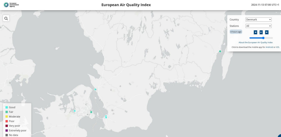
Figur 2.6. EEA luftkvalitetsindeks for København. Måledata stammer fra H.C. Andersens Boulevard og prognose data fra CAMS ( https://www.eea.europa.eu/en/analysis/maps-and-charts/index ).
