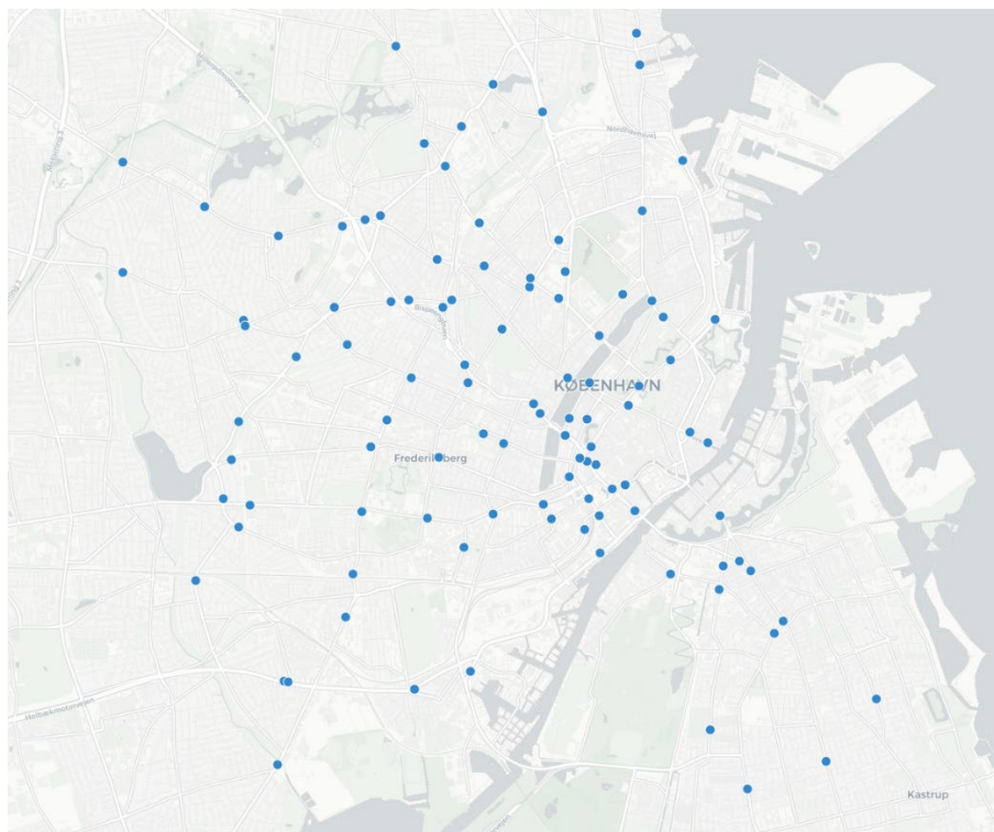
Figur 3.1. Placering af 103 lokationer, som indgår i prognose- og varslingssystem.
