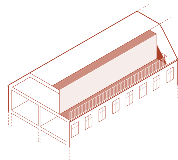
Principskitse af lodret facadeparti i københavertag.
