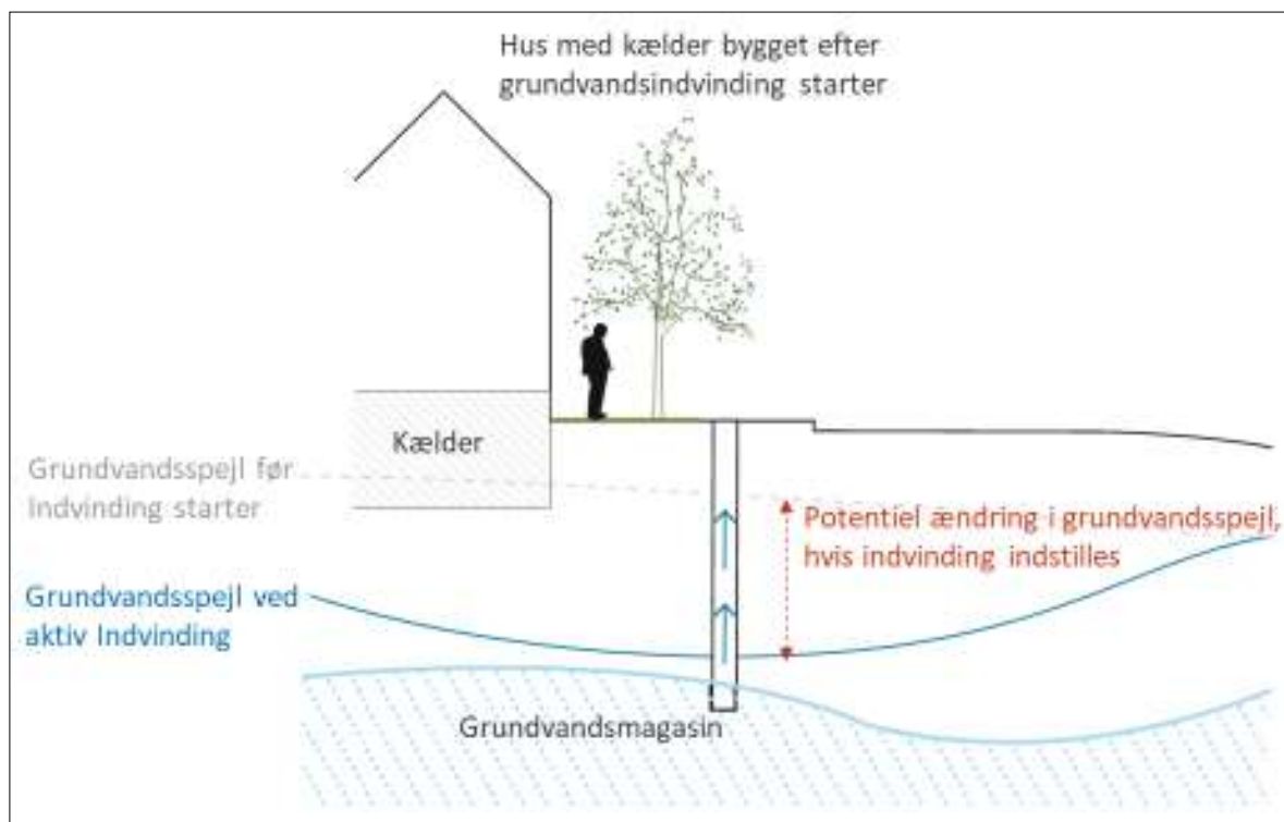
Figur 3-2. Påvirkning af grundvandsspejlet ved indstilling eller reduktion af grundvandsindvinding.
