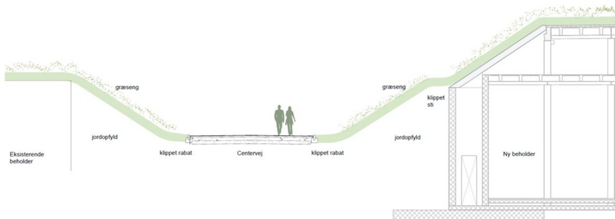
Figur 2 Skematisk tværsnit af beholderkonstruktion ved opbevaring af drikkevandet i "beholder i beholder".
