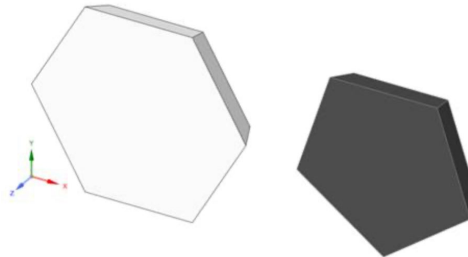
Polygonmoduler bestående af 5- og 6-kant med kantlængder på 70 cm
