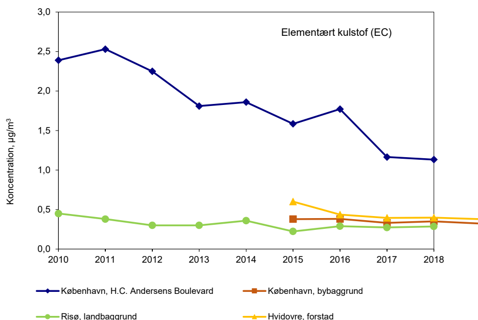
Figur 3.2. Udviklingstendens for årsmiddelkoncentrationen af elementært kulstof siden opstart af målingerne i 2010 (Ellermann et al., 2020).
