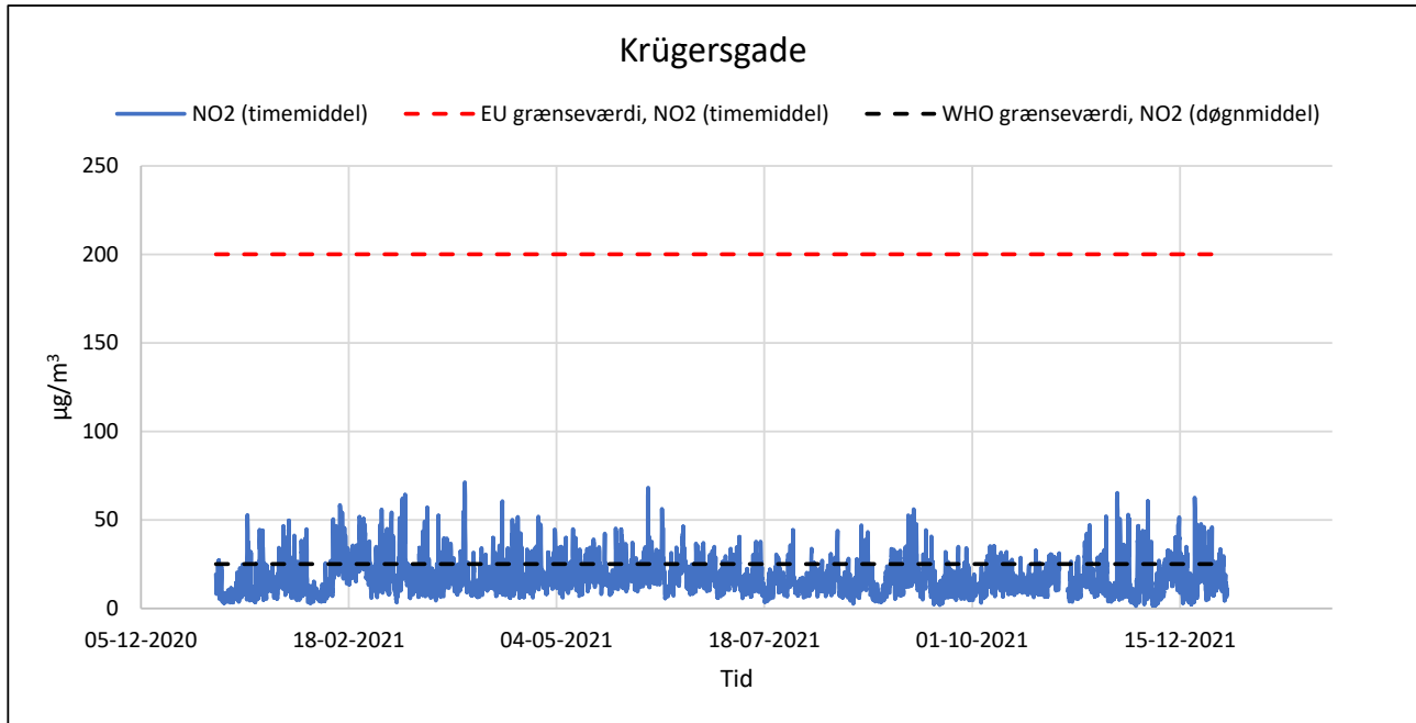
Figur 53. Timemiddelværdier for NO 2 på Krügersgade.
