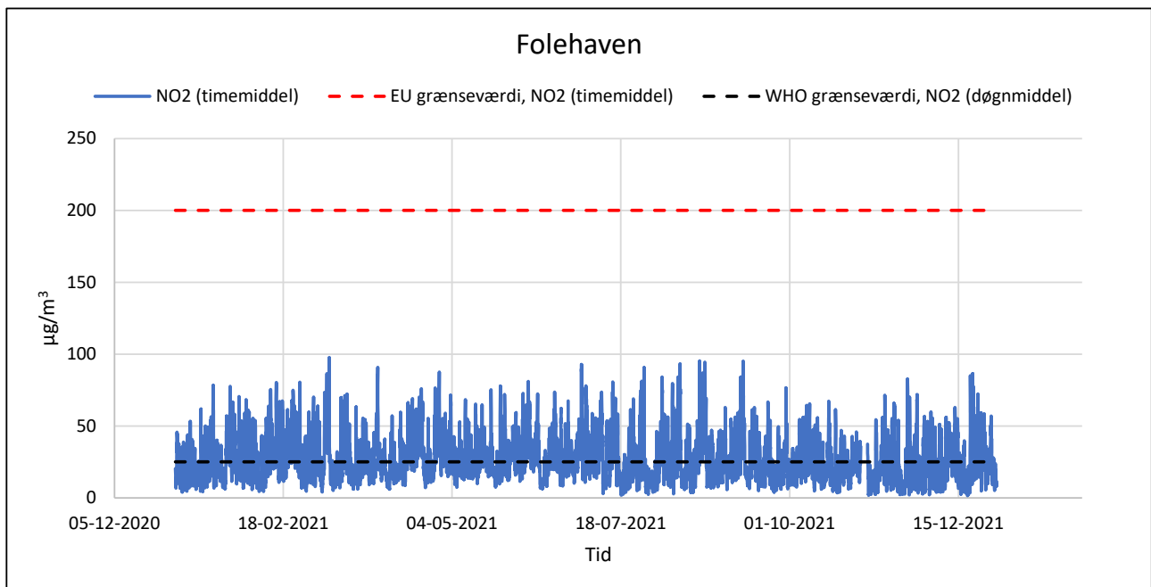
Figur 56. Timemiddelværdier for NO 2 på Folehaven.
