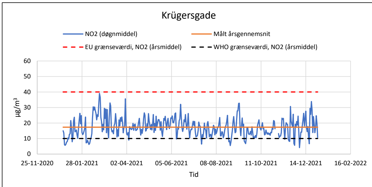
Figur 20. Døgnmiddelværdier samt målt årgennemsnit for NO 2 på Krügersgade. Den røde og sorte stiplede linje angiver henholdsvis EU's grænseværdi samt WHO's vejledende grænseværdi for den gennemsnitlige koncentration af NO 2 over et år.
