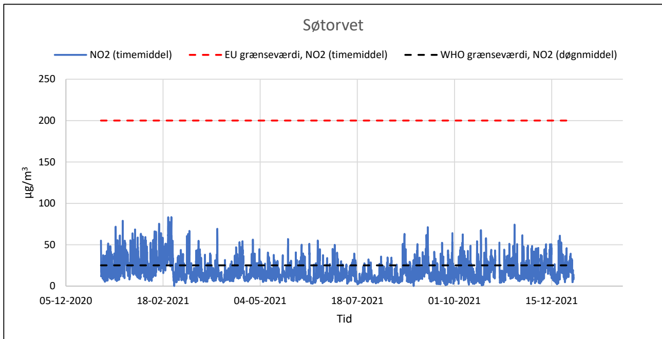
Figur 54. Timemiddelværdier for NO 2 på Søtorvet.
