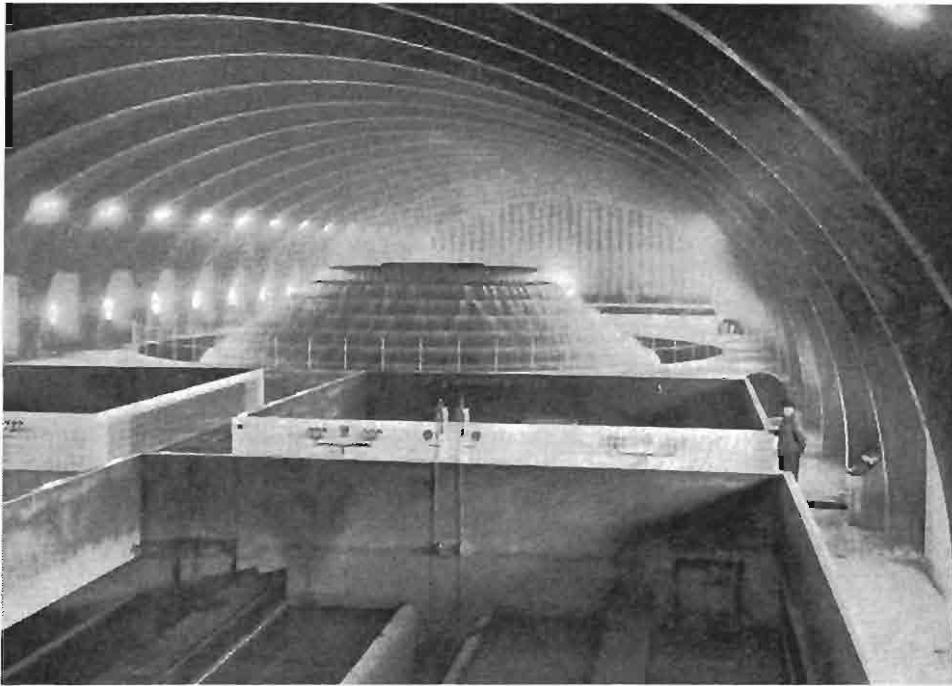
Slangerupværket (iltningsanlægget).
