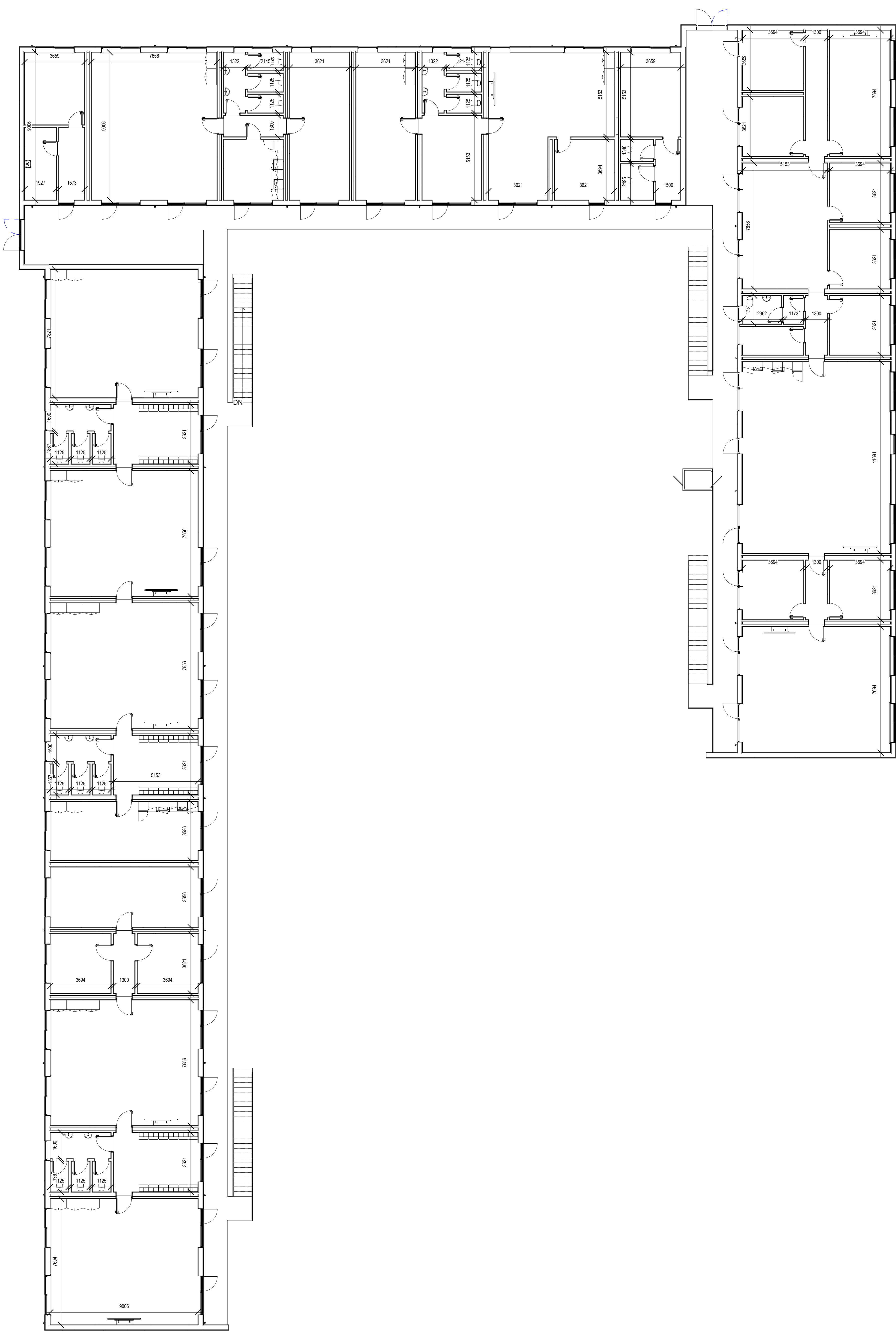
1 1. Sal Målsat 1 : 115
