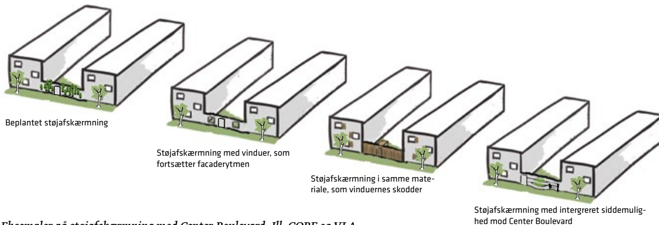
Eksempler på støjafskærmning mod Center Boulevard. Ill. COBE og VLA
