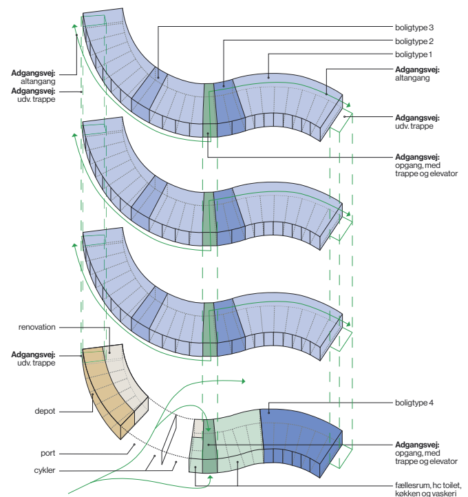
Funktions diagram
