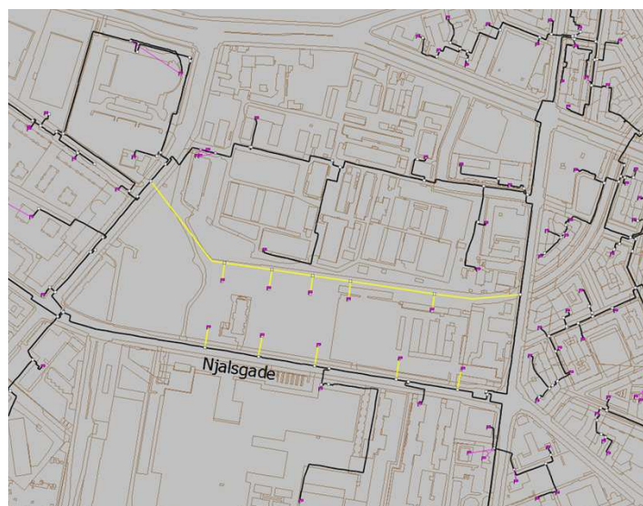
Figur 3 Udbygget ledningsnet for Faste Batteri III
