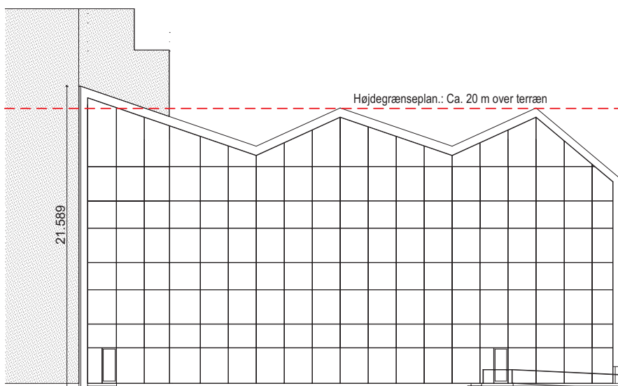
Eksisterende bygning
