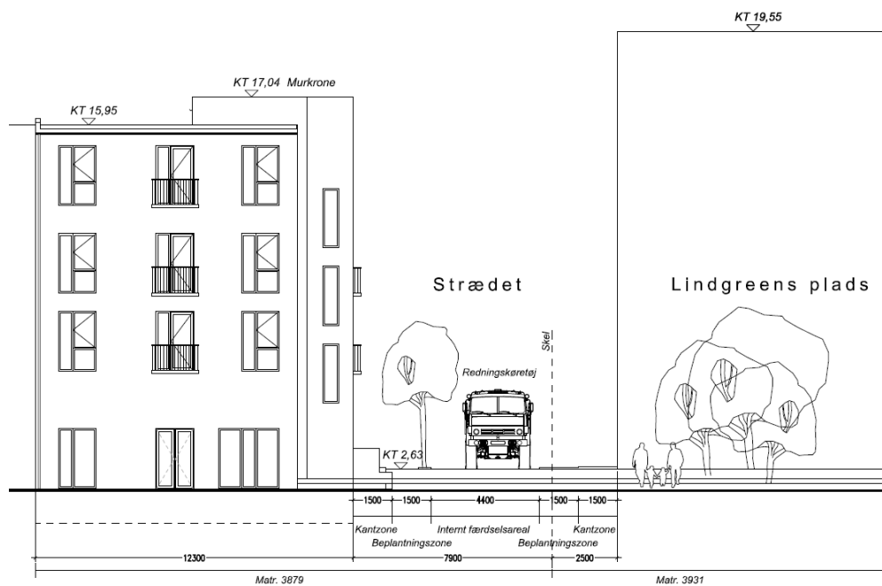
Fremtidigt profil - 'Strædet'
