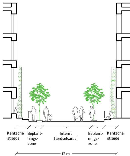
Tegning nr. 3a fra lokalplan nr. 550 - vejsnit (Snit B - udformning af strædet)
