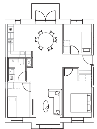
4 værelses familiebolig
