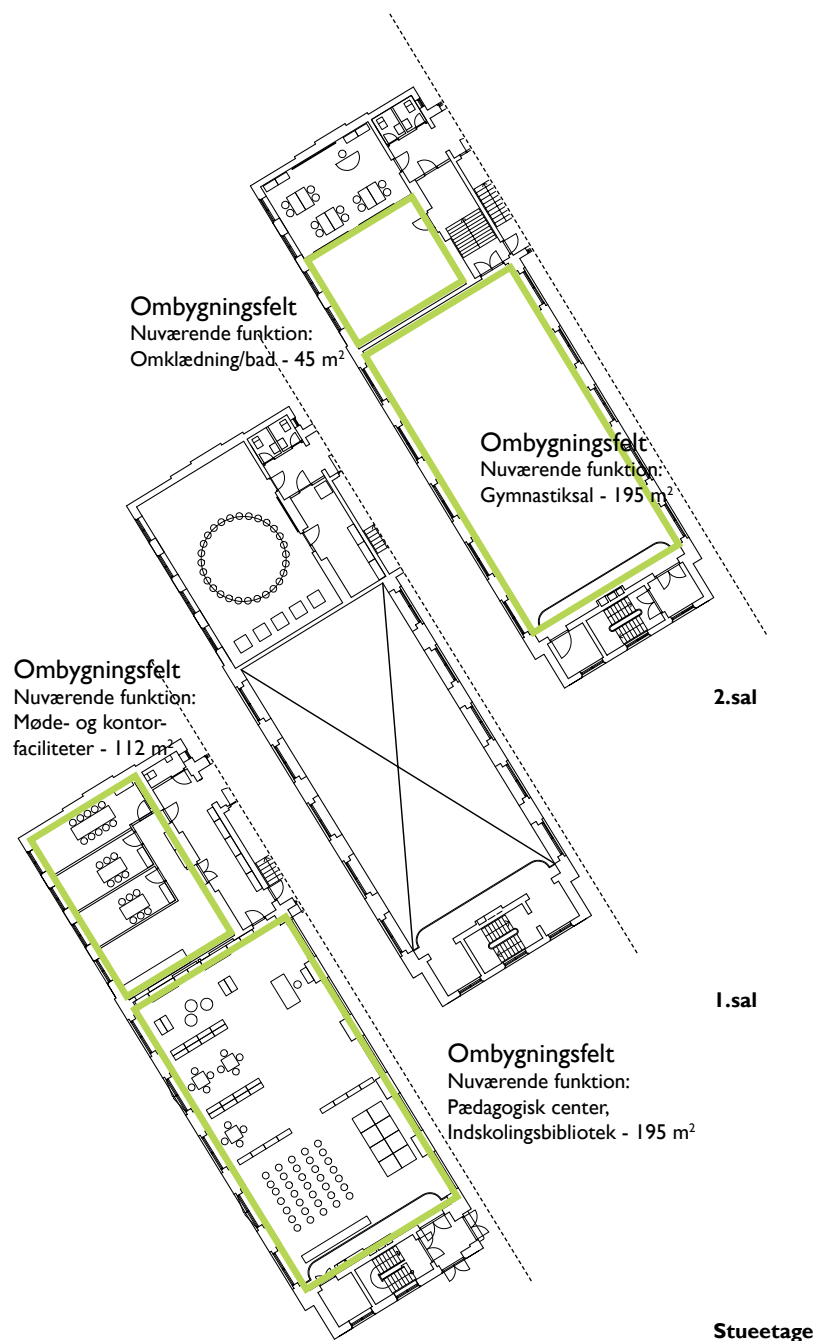
Plantegninger af Vestfløjen og de 4 lokaler der ombygges samt deres nuværende funktioner.
