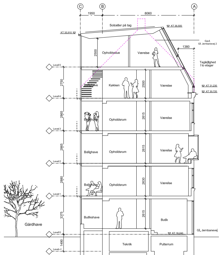
Snit - 1:200. Ill. af Domus Arkitekter.
