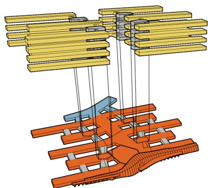
Figur 1: Princip for bebyggelse indenfor byggeområde 2. Længebygninger (vist med gul). Base (vist med rød). Bygning i nordlige landskabsrum (vist med blå). Forbindelsesbygninger og trappe/elevatortårne (vist med grå).
