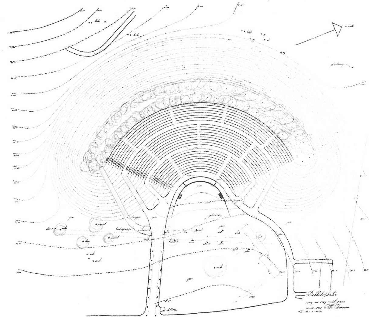
C.TH. Sørensens tegning af Bellahøj Friluftsscene, dateret 28.12.1951. Udførelsen af teatret er stort set gennemført som tegningen.
