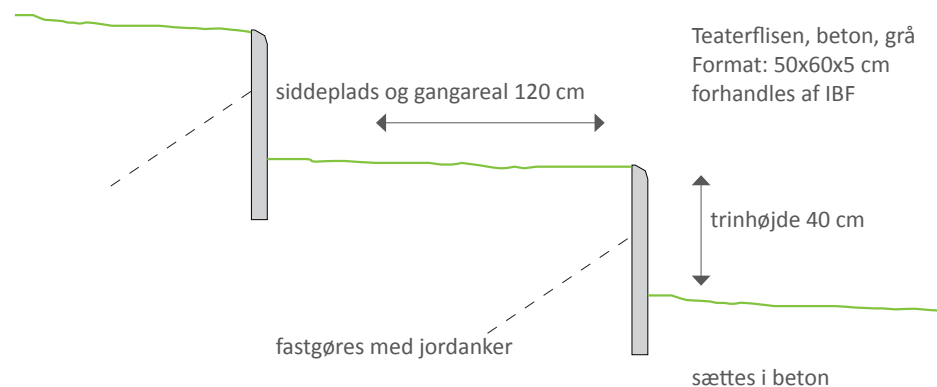
Principielt snit i betonkanter/siddekanter
