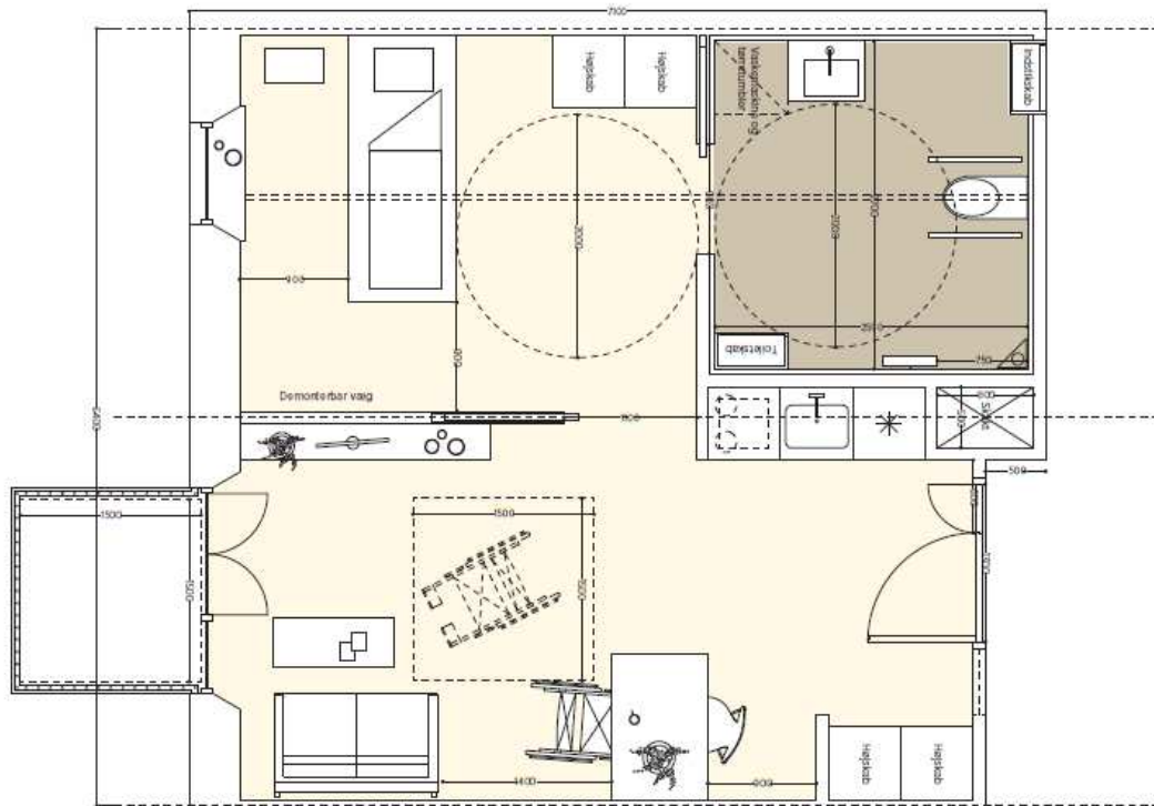
Figur 6: Plantegning af bolig
