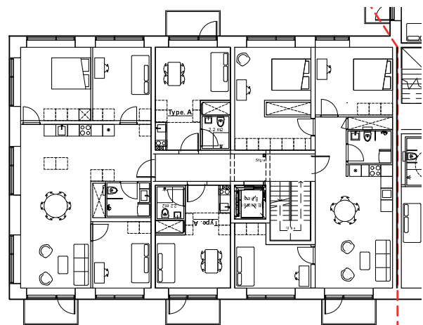
Boligplaner 1-3 sal
