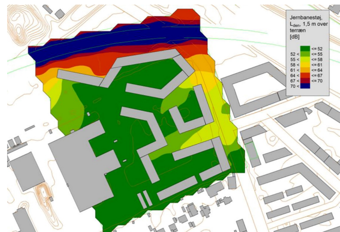
Jernbanestøj 1,5 m over terræn. Illustration Gade & Mortensen.
