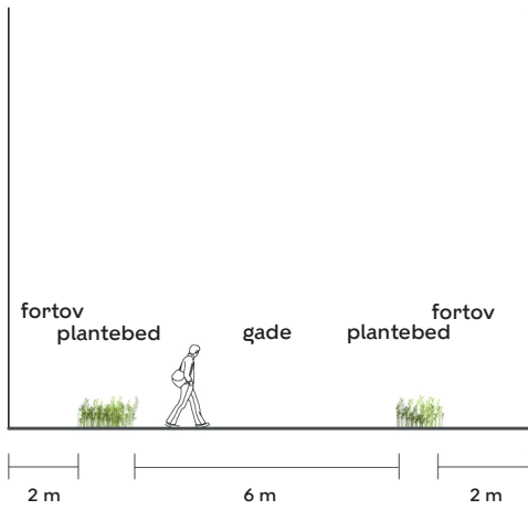
Snit A-A
