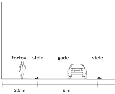
Snit B-B
