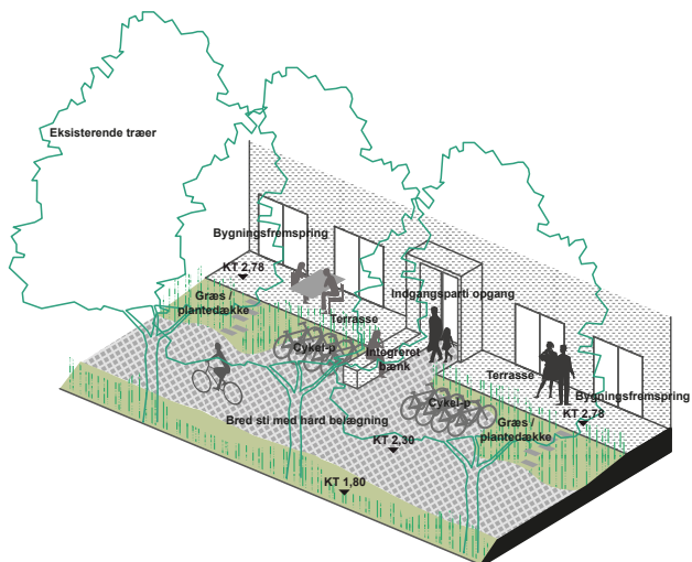
Kantzone d mod 'Poppelstien'
