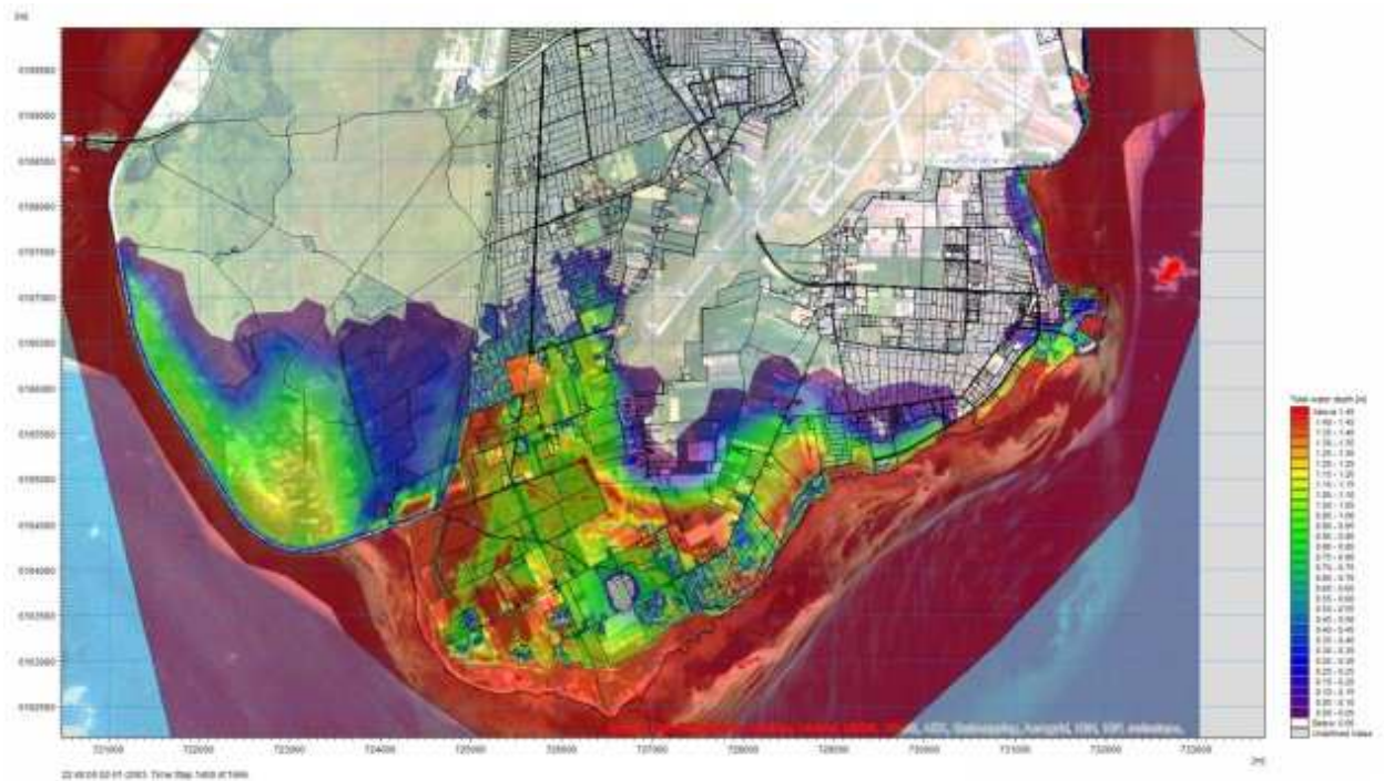
Figur 6: Oversvømmelser som følge af 100 års stormflod i 2050 ved Sydamer (fra rapporten Højvandsbeskyttelse af Sydamer udarbejdet af NIRAS for Dragør og Tårnby Kommune og Kalvebod Pumpedigeaug).
