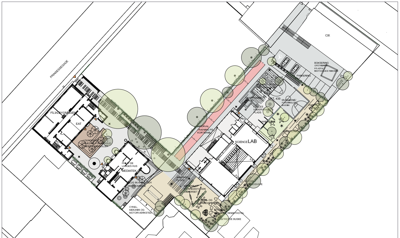
Situationsplan. (Ill.: Rubow Arkitekter).
