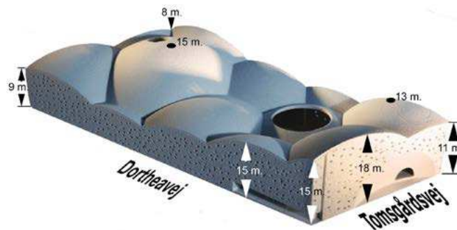
Figur 1: Skitse, der principielt illustrerer bygningen udformet med et antal kuglehvæl. Maksimale højder er markeret på tegningen (Illustration Henning Larsen Architects)
